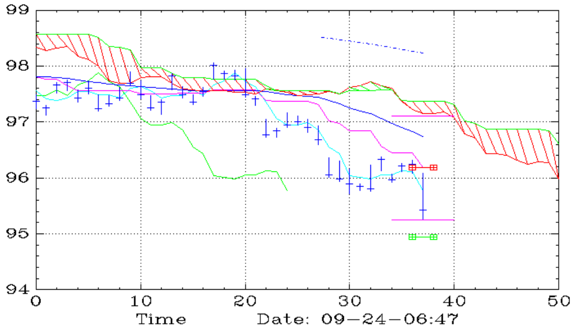
AGG (Daily,Ichimoku)
