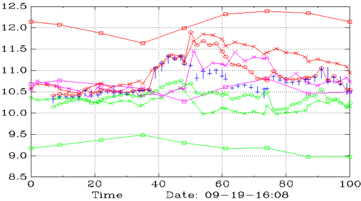
AI (Daily,90,60)
