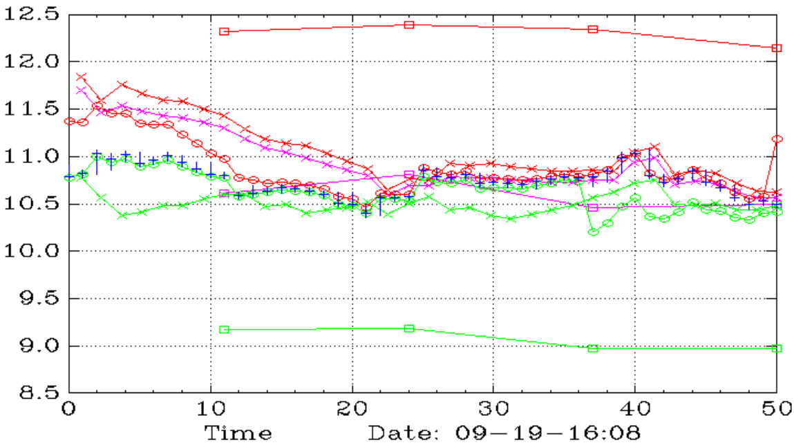
AI (Daily,45,30)
