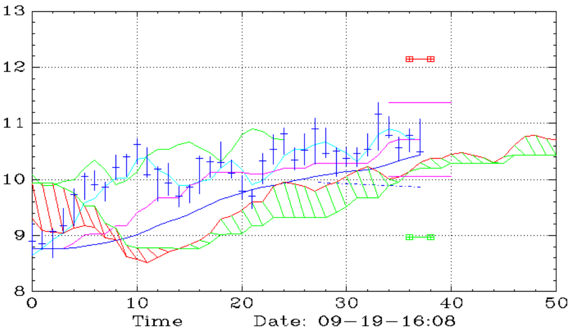
AI (Daily,Ichimoku)
