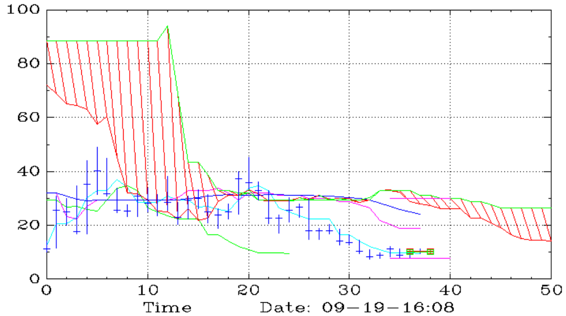
AI (Monthly,Ichimoku)
