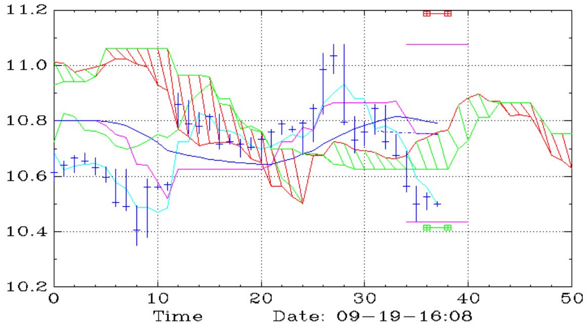
AI (30,Ichimoku)
