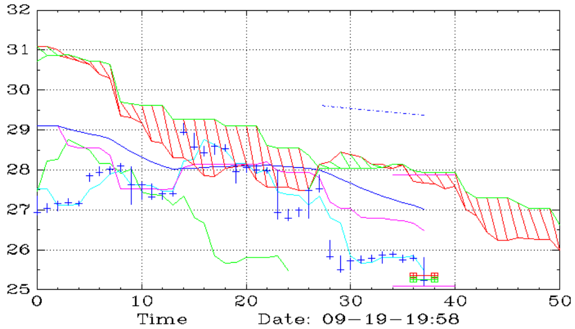
AMDD (90,Ichimoku)
