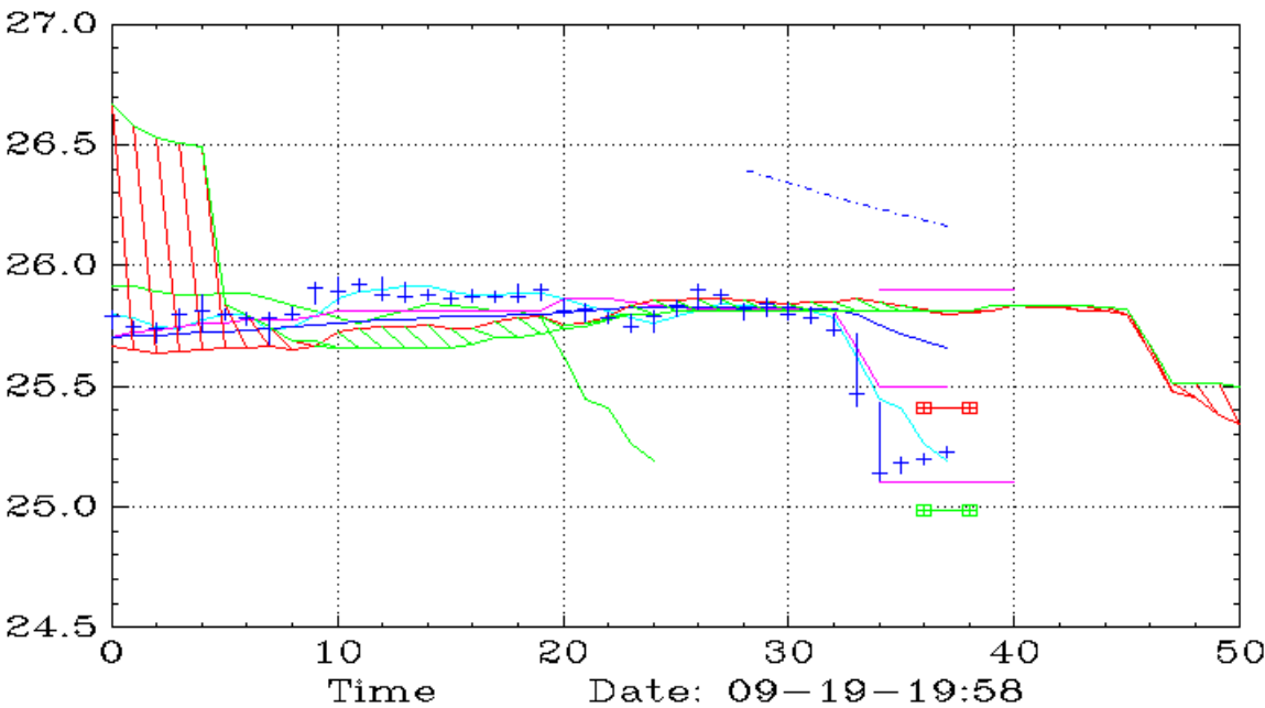
AMDD (10,Ichimoku)
