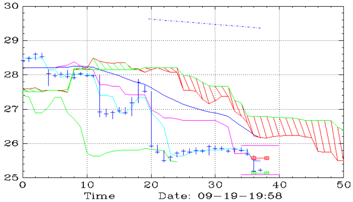
AMDD (45,Ichimoku)
