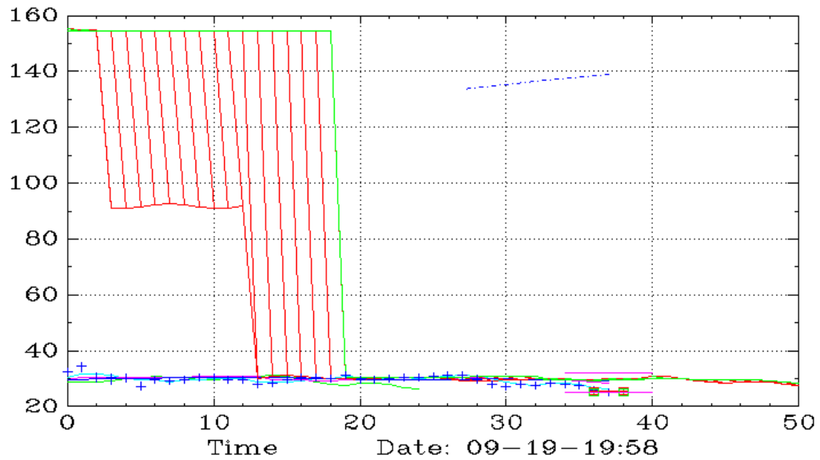
AMDD (Daily,Ichimoku)
