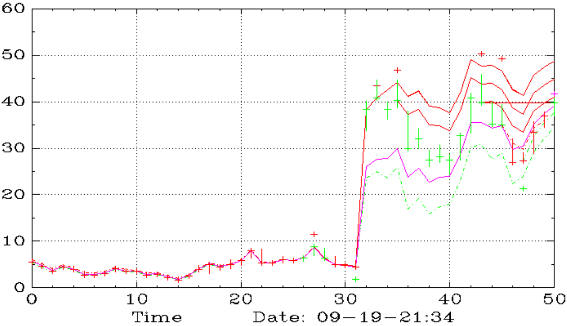
AXTU (Daily,SAR)
