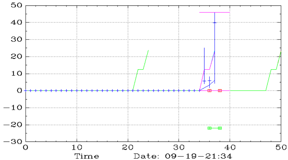
AXTU (Monthly,Ichimoku)
