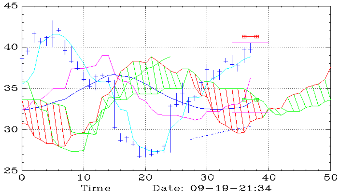
AXTU (90,Ichimoku)
