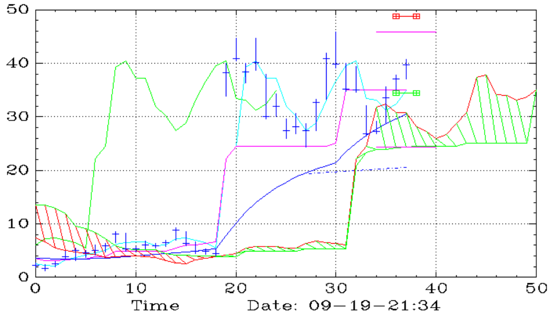
AXTU (Daily,Ichimoku)
