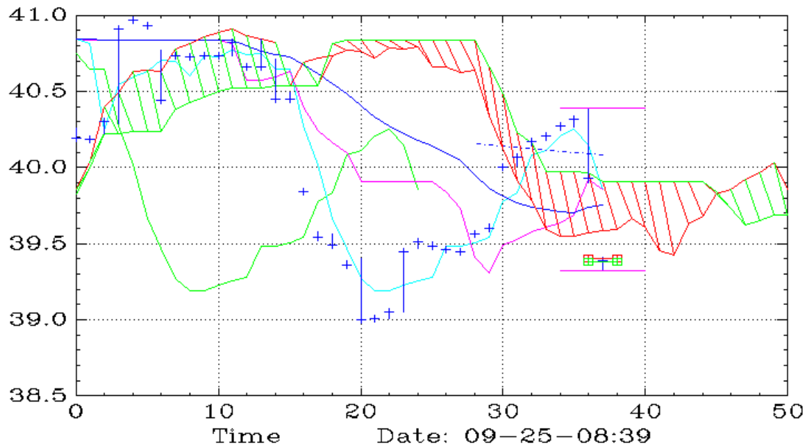
BKF (10,Ichimoku)
