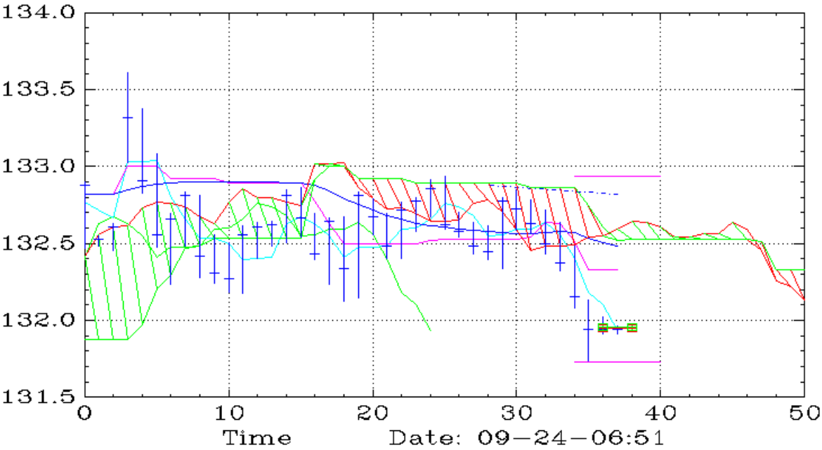
C (10,Ichimoku)
