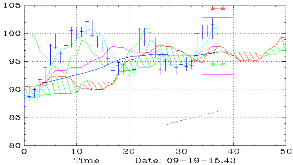
CIBR (Daily,Ichimoku)
