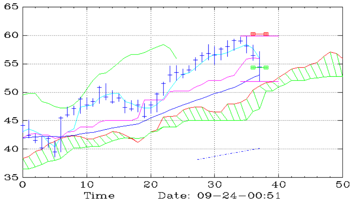
CLMT (Daily,Ichimoku)
