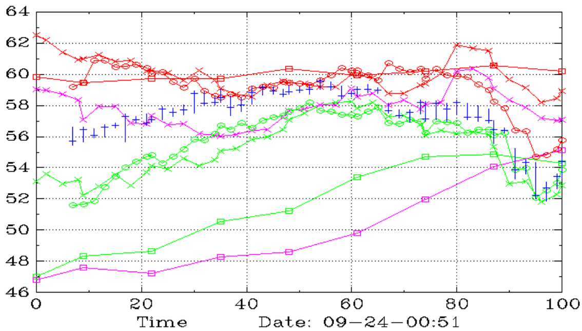
CLMT (Daily,90,60)
