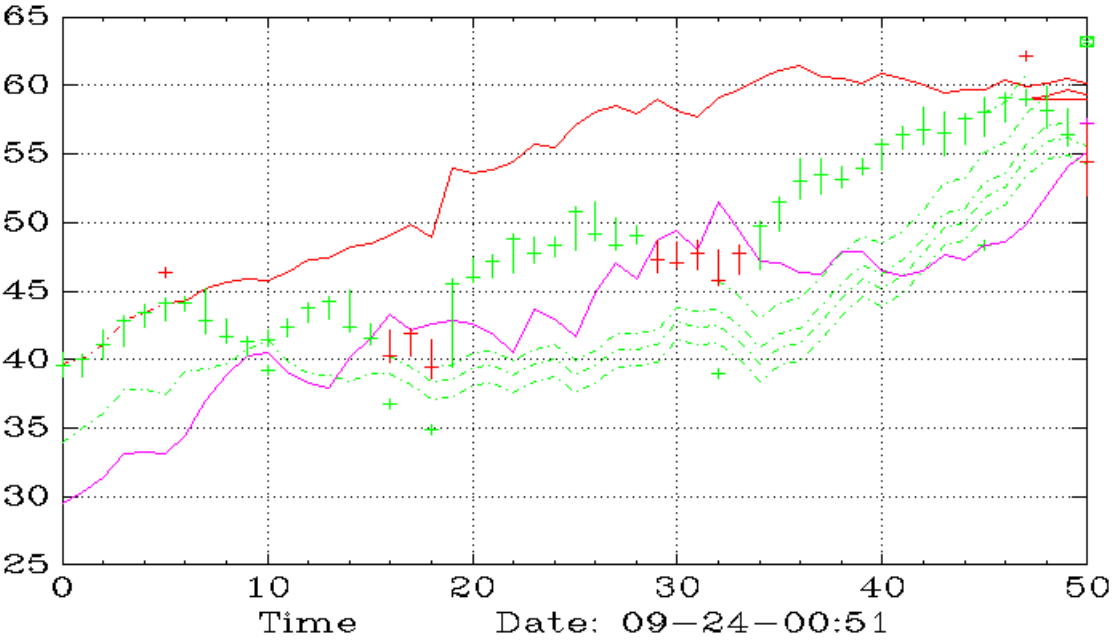
CLMT (Daily,SAR)
