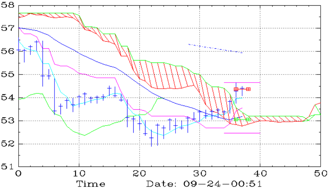
CLMT (10,Ichimoku)
