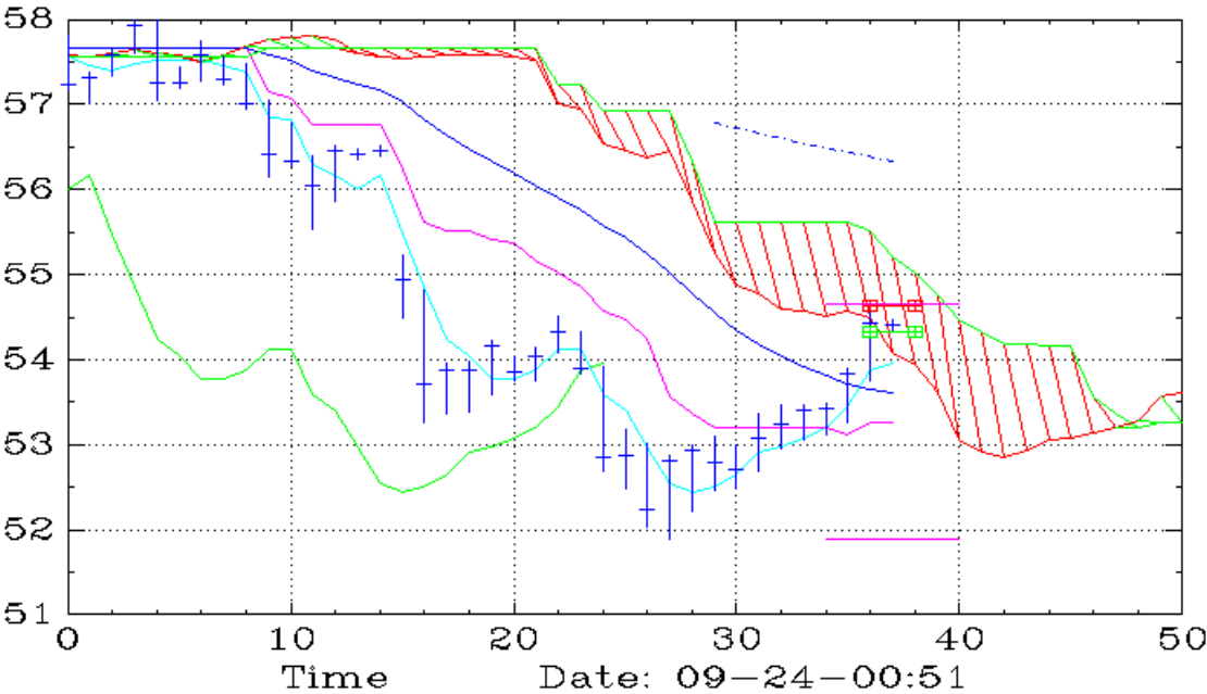
CLMT (15,Ichimoku)
