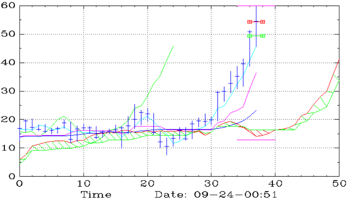
CLMT (Monthly,Ichimoku)
