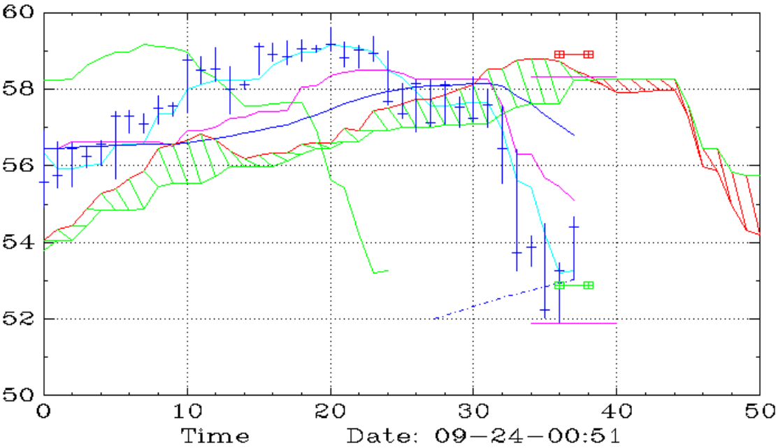
CLMT (90,Ichimoku)
