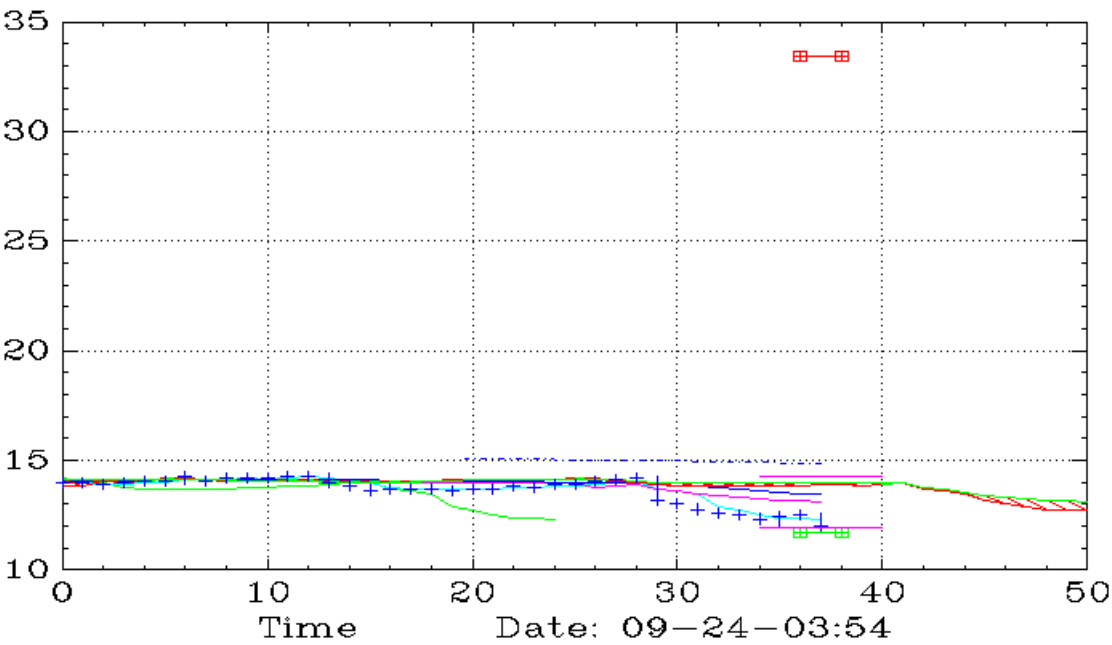
CLYM (45,Ichimoku)
