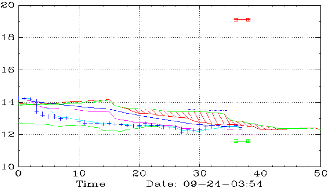
CLYM (10,Ichimoku)
