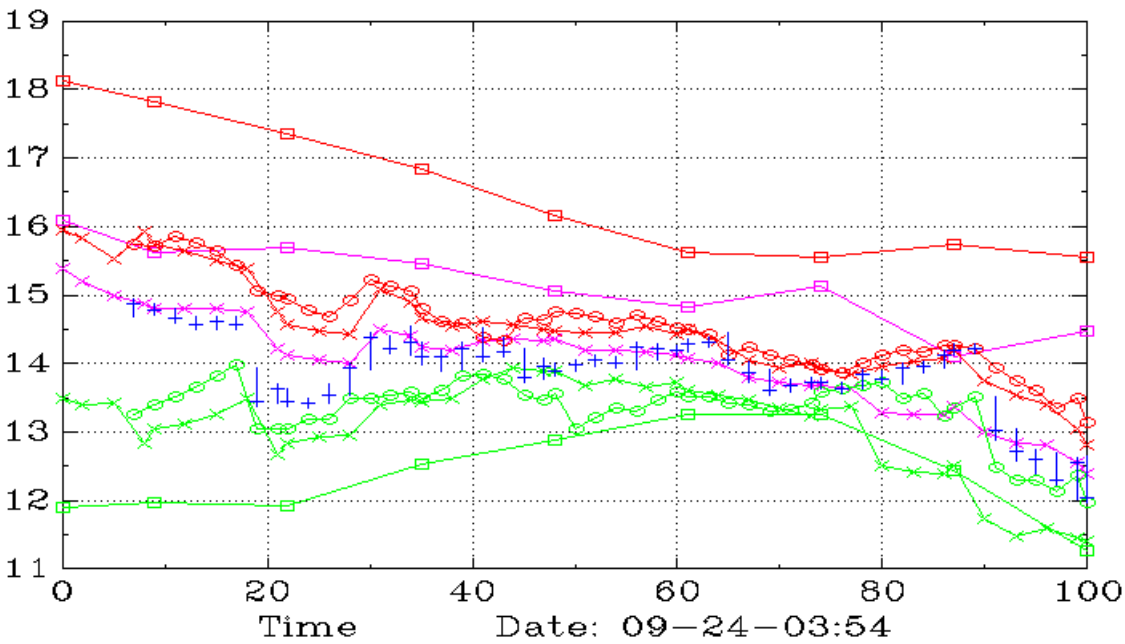
CLYM (Daily,90,60)
