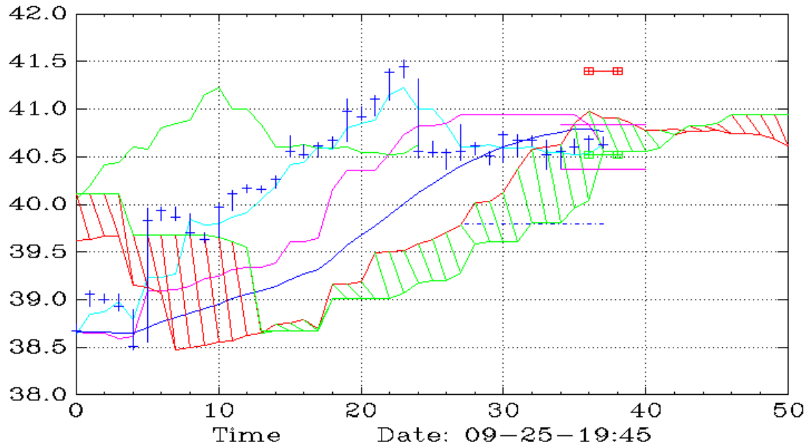
CPER (90,Ichimoku)
