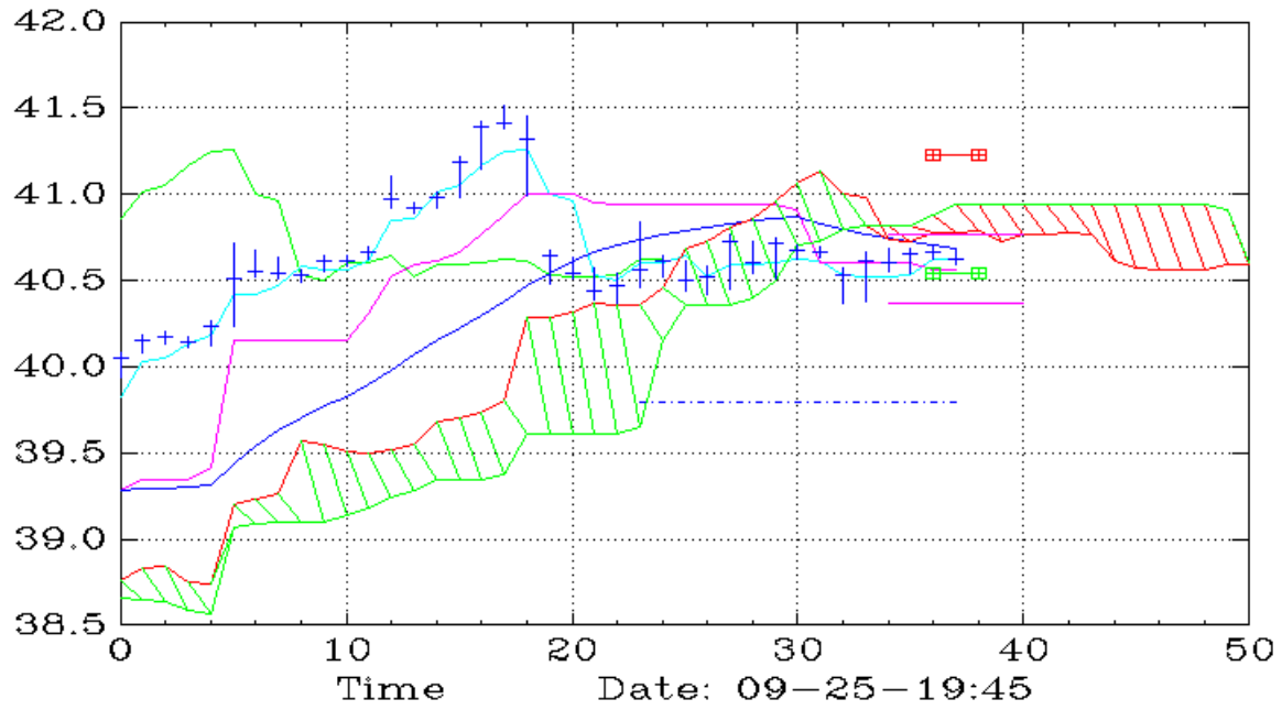
CPER (60,Ichimoku)
