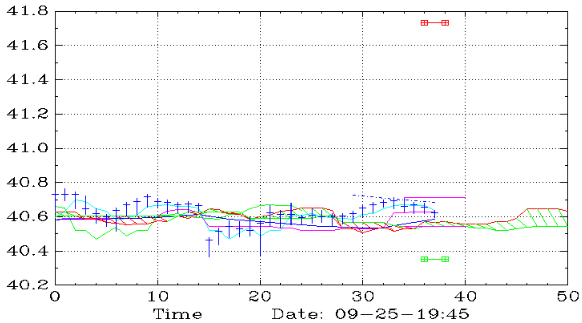
CPER (15,Ichimoku)
