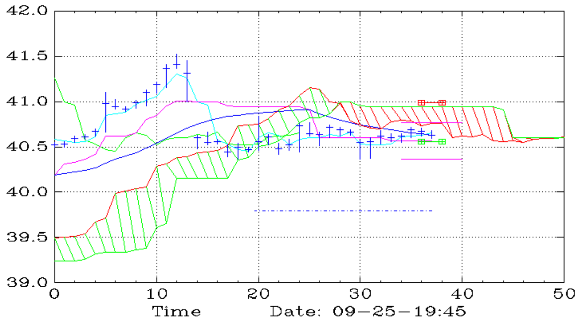
CPER (45,Ichimoku)
