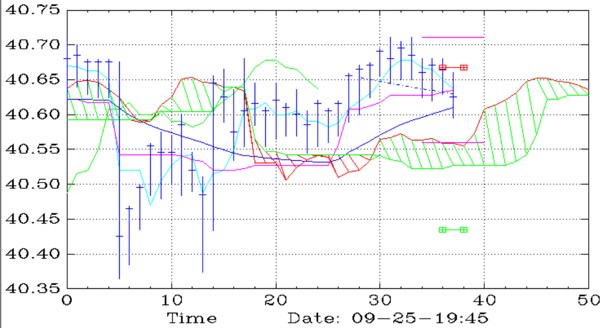
CPER (10,Ichimoku)
