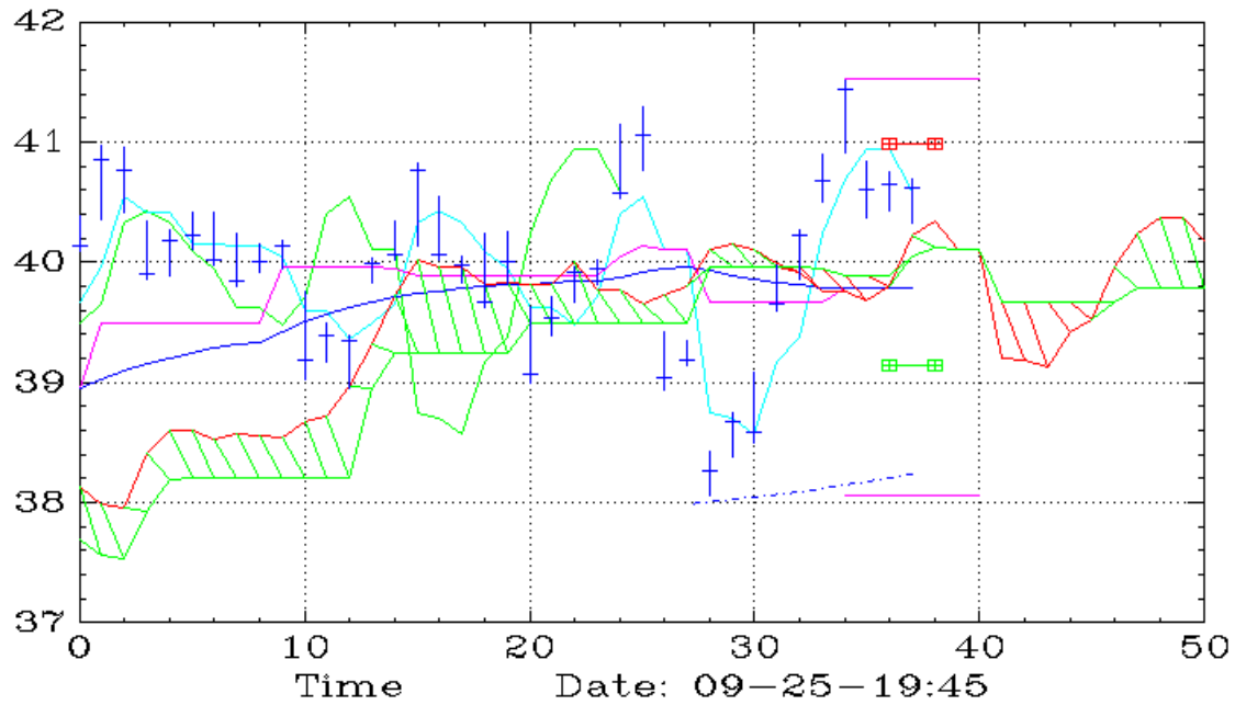
CPER (Daily,Ichimoku)
