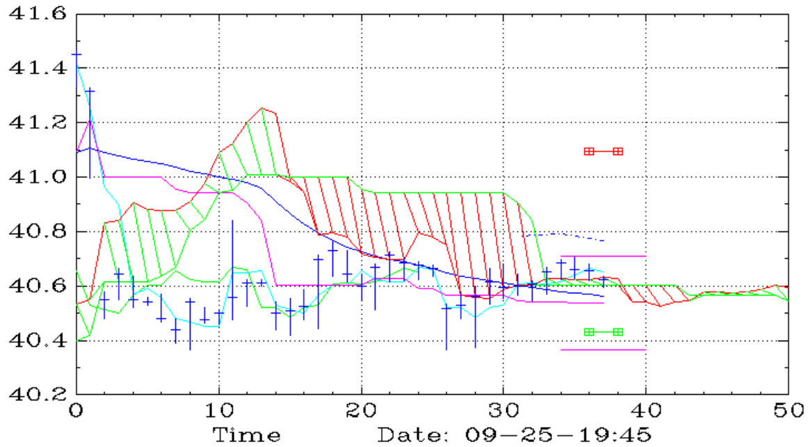
CPER (30,Ichimoku)
