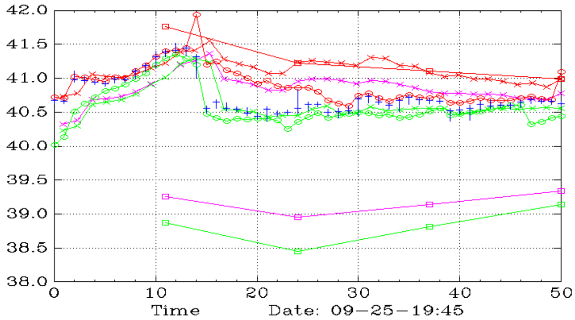
CPER (Daily,45,30)
