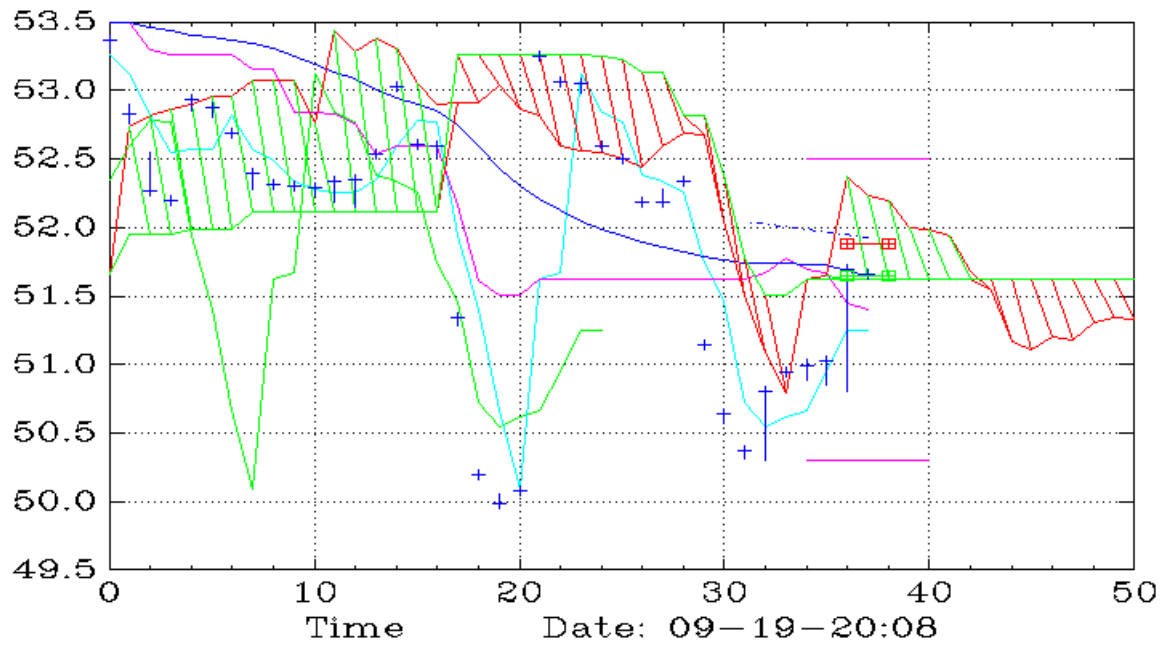
CSCL (30,Ichimoku)
