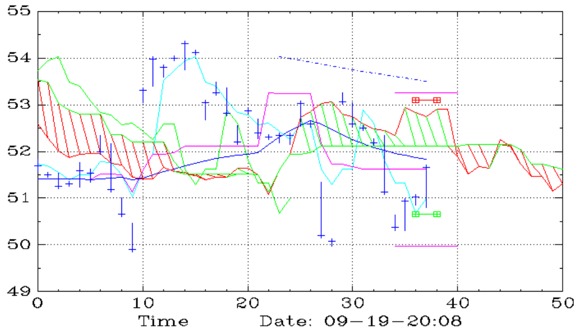
CSCL (60,Ichimoku)
