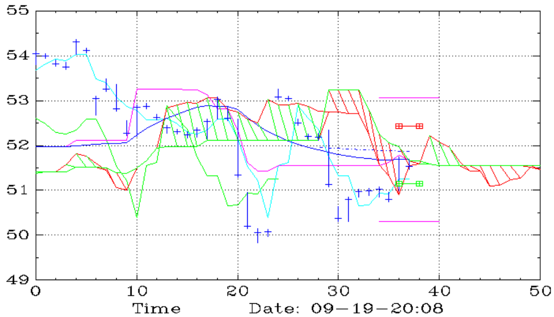
CSCL (10,Ichimoku)
