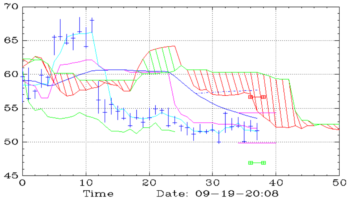
CSCL (Daily,Ichimoku)
