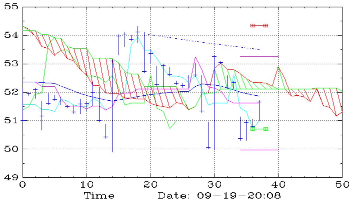
CSCL (45,Ichimoku)
