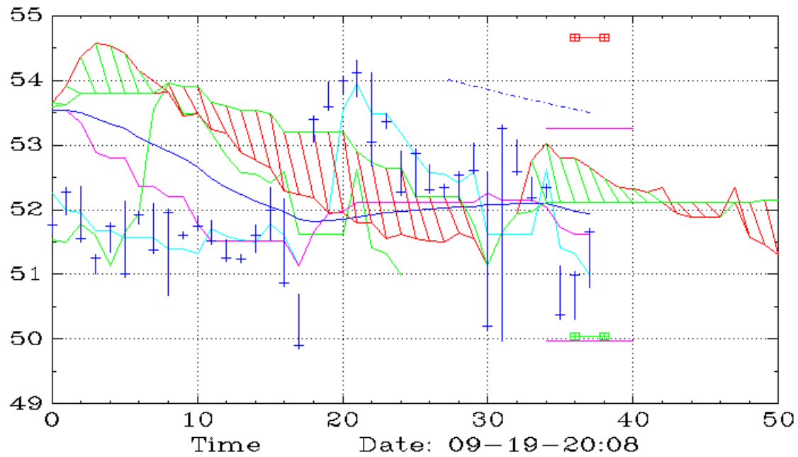
CSCL (90,Ichimoku)
