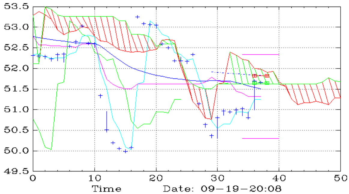
CSCL (15,Ichimoku)
