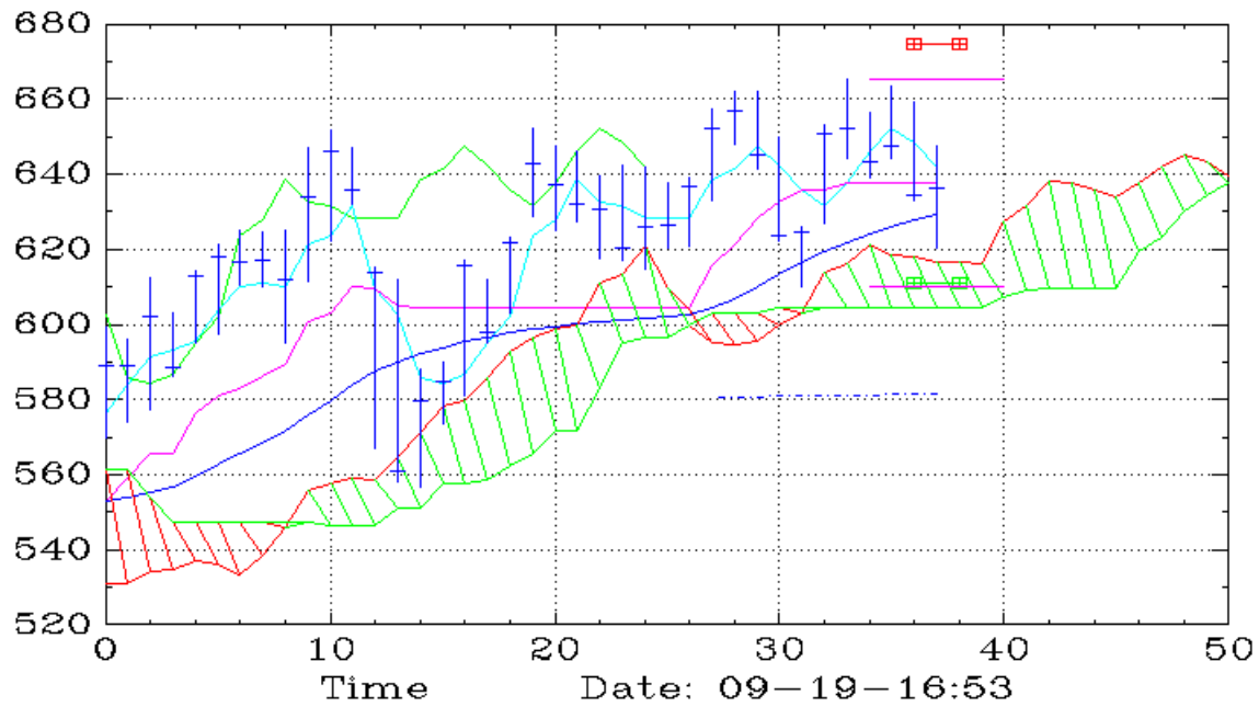
DDS (Daily,Ichimoku)
