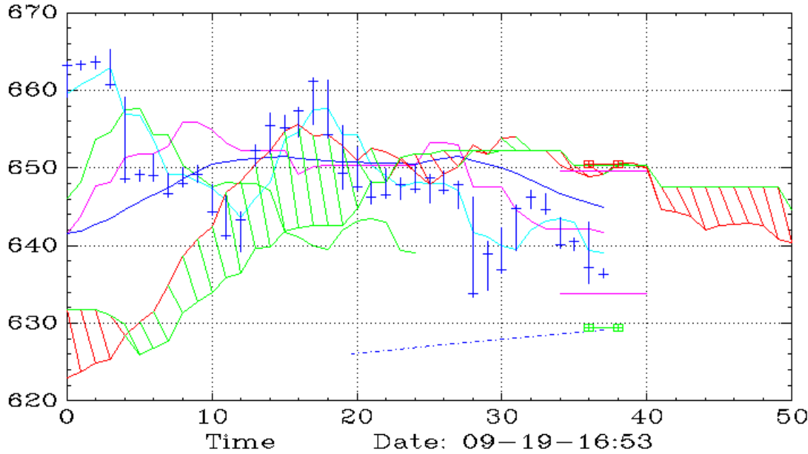
DDS (45,Ichimoku)
