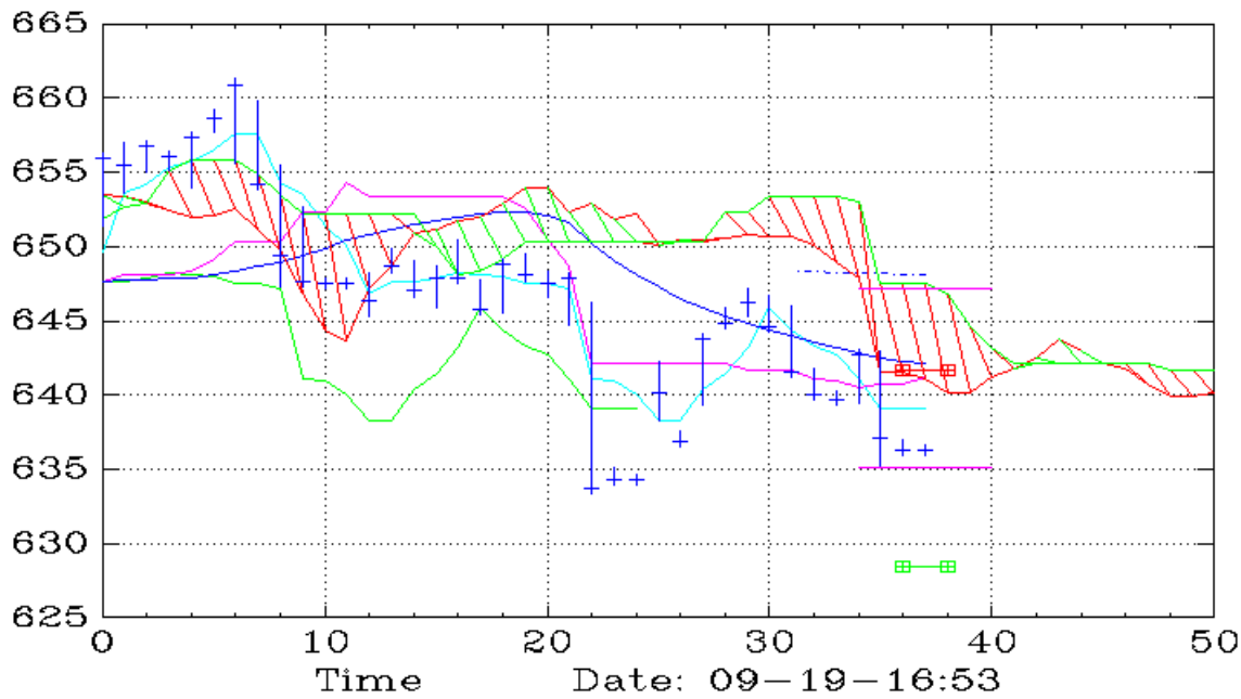
DDS (30,Ichimoku)
