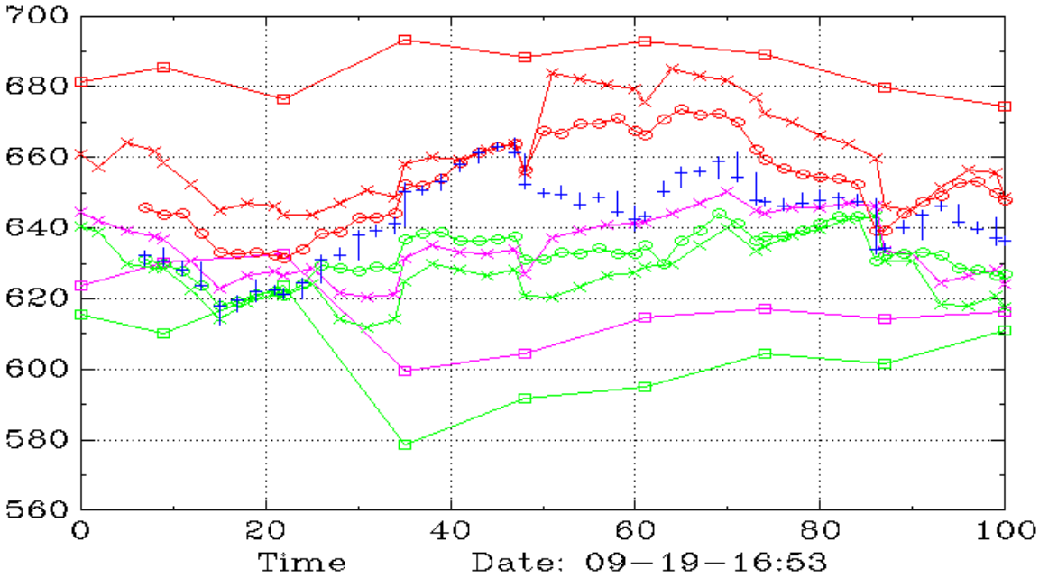
DDS (Daily,90,60)
