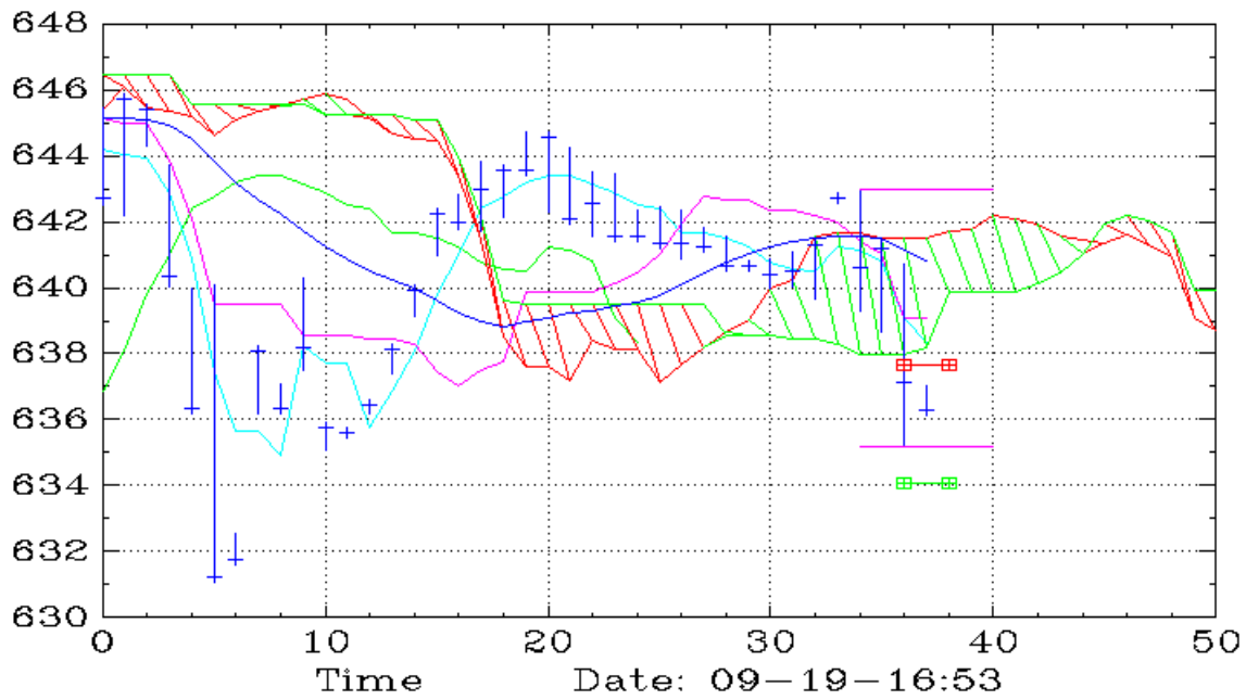
DDS (10,VAP_Ichimoku)
