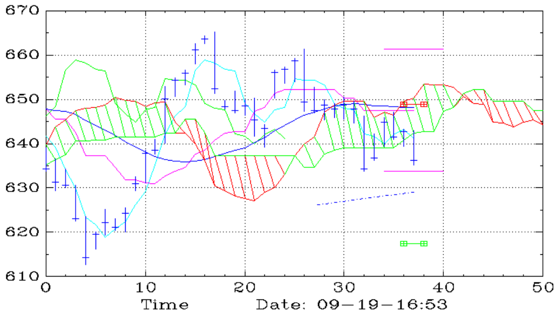
DDS (90,Ichimoku)
