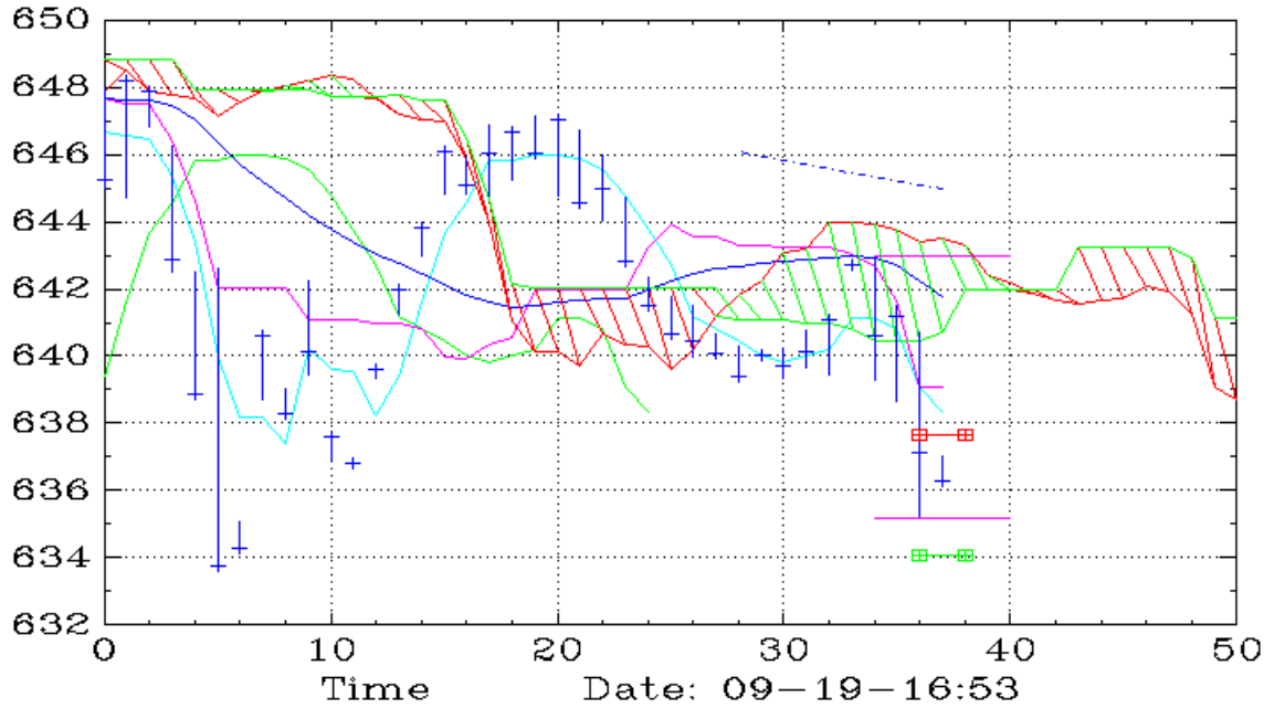
DDS (10,Ichimoku)
