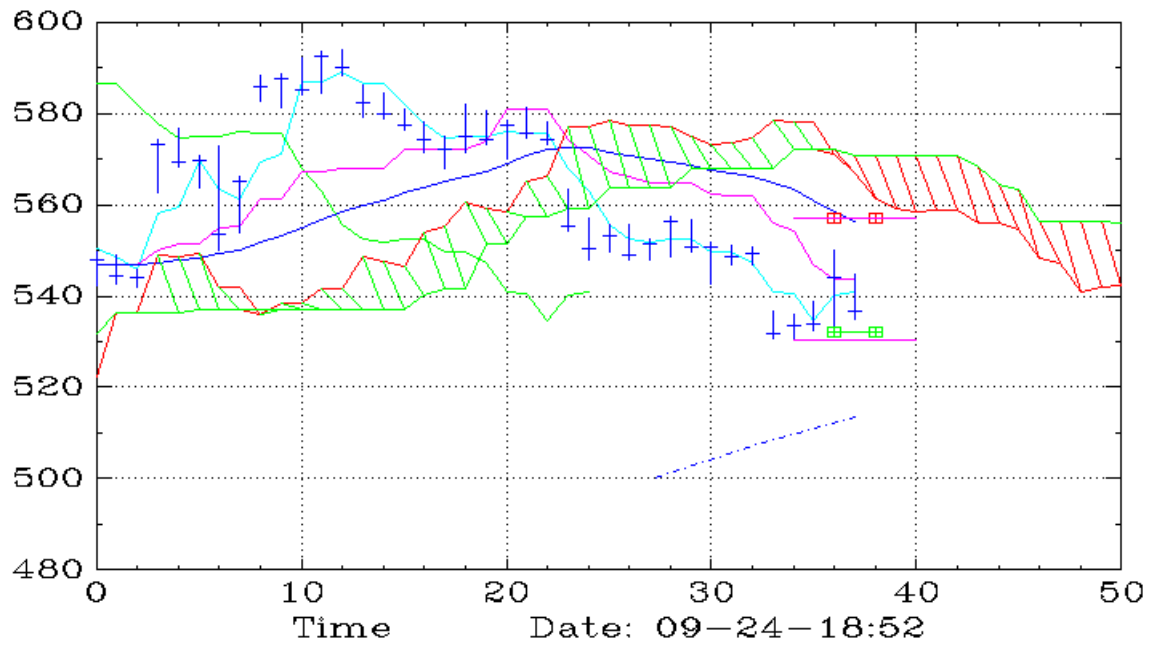
DELL (90,Ichimoku)
