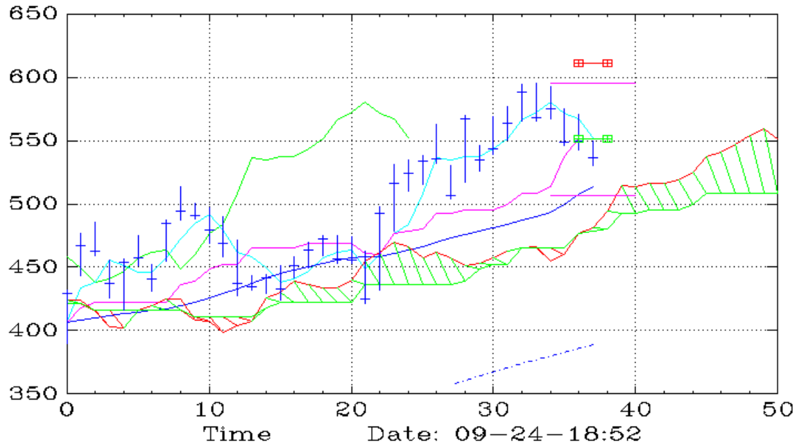
DELL (Daily,Ichimoku)
