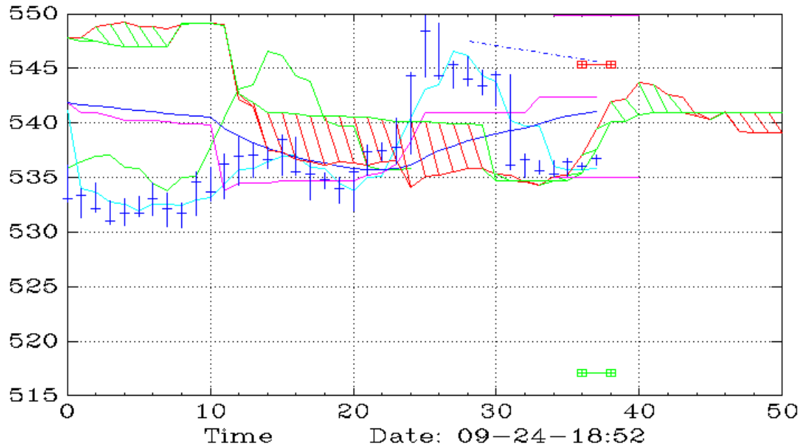
DELL (10,Ichimoku)
