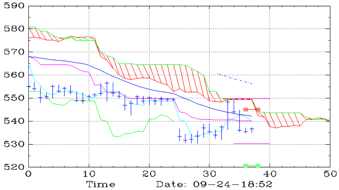
DELL (30,Ichimoku)
