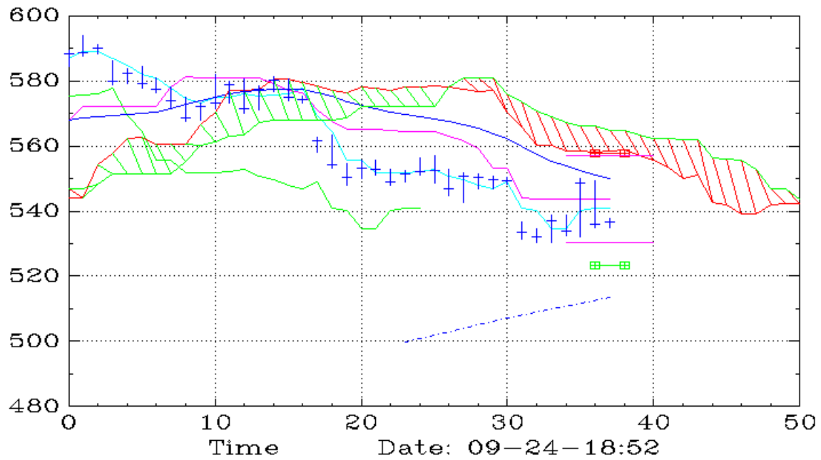
DELL (60,Ichimoku)
