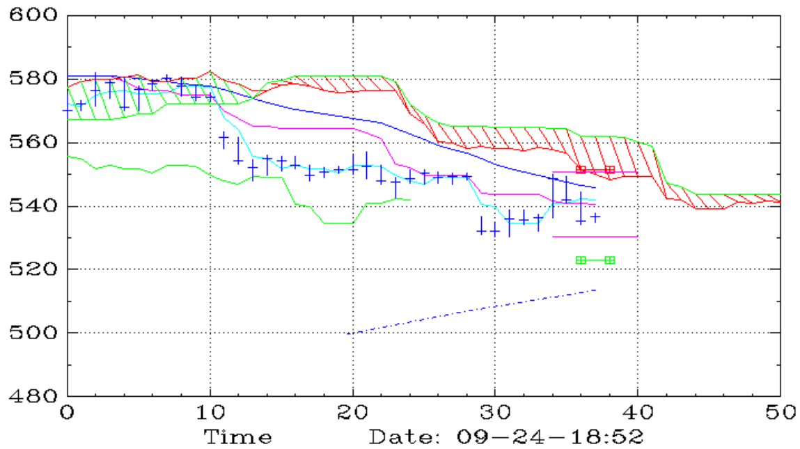
DELL (45,Ichimoku)
