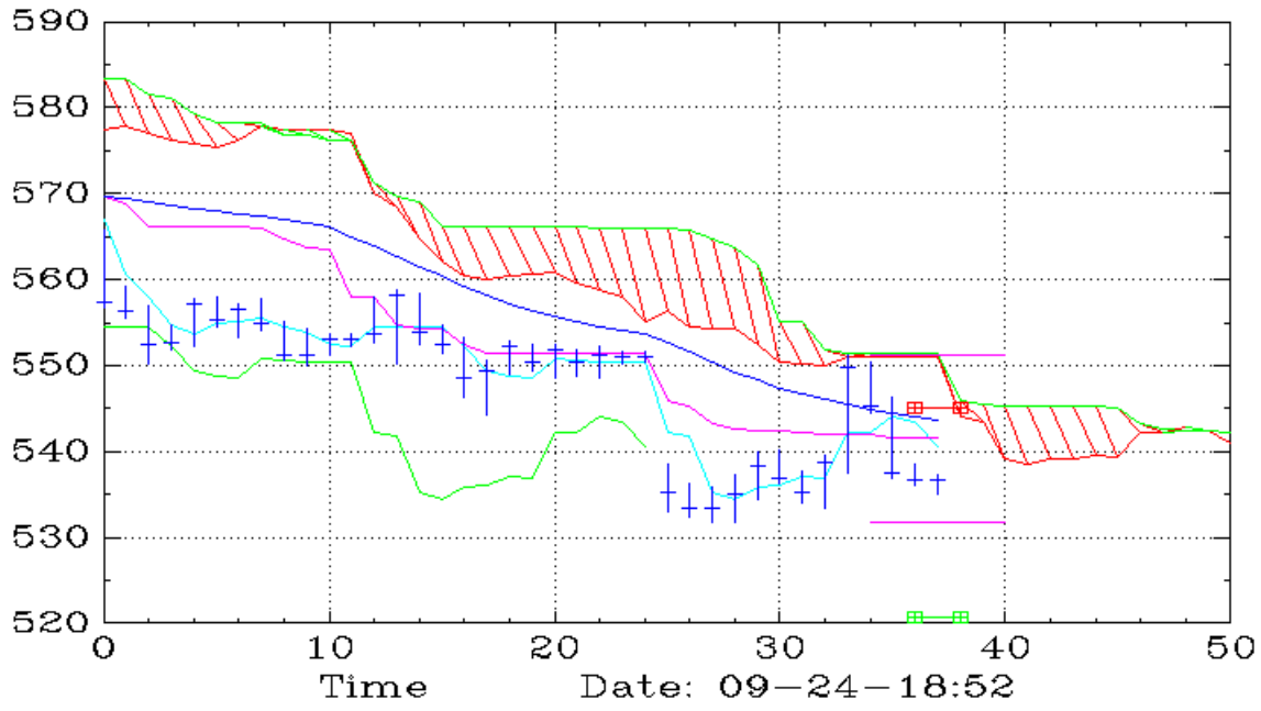
DELL (30,VAP_Ichimoku)
