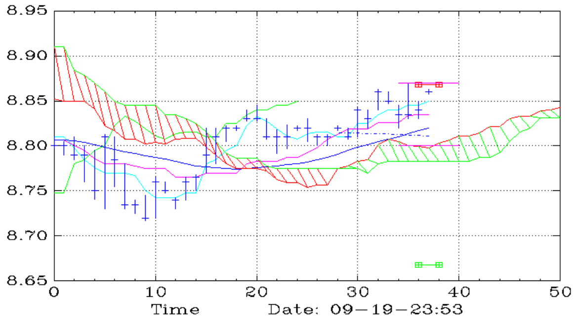
ERY (10,Ichimoku)
