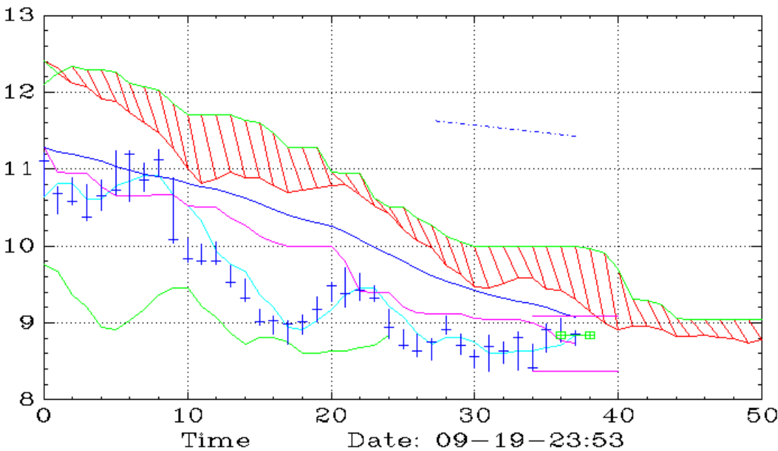
ERY (Daily,Ichimoku)
