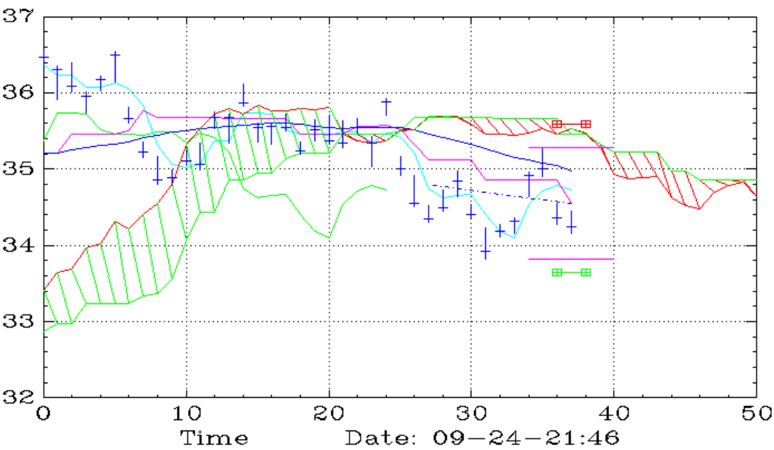
FXI (Daily,Ichimoku)
