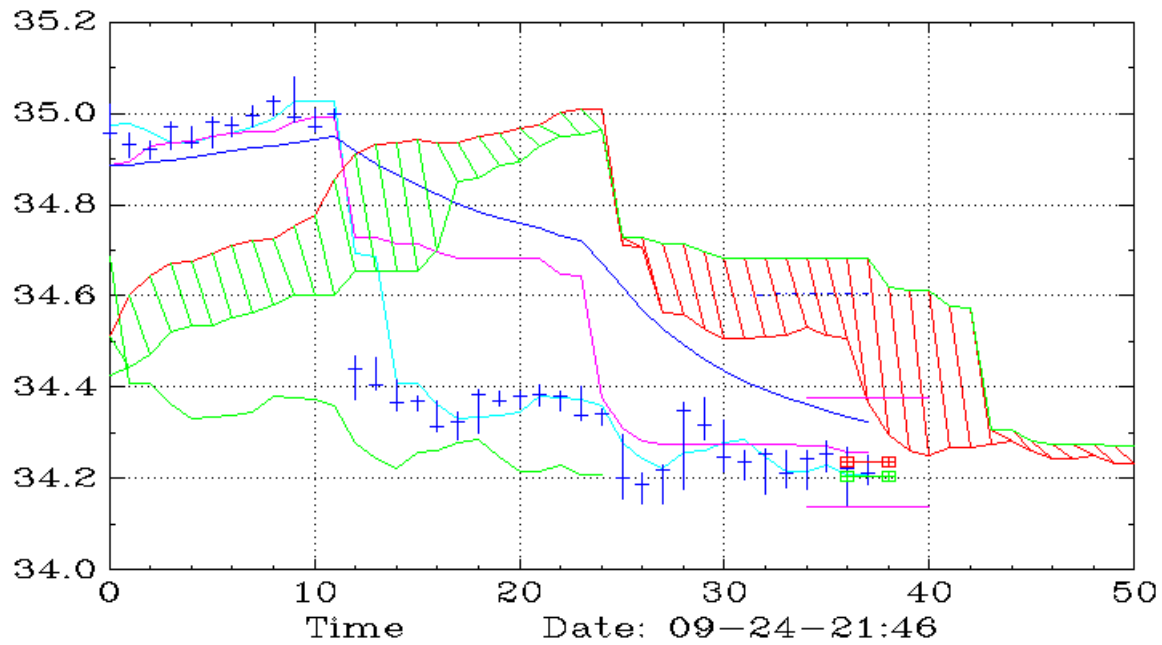
FXI (30,Ichimoku)
