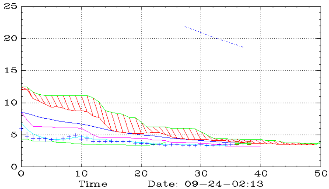
GNPX (Daily,Ichimoku)
