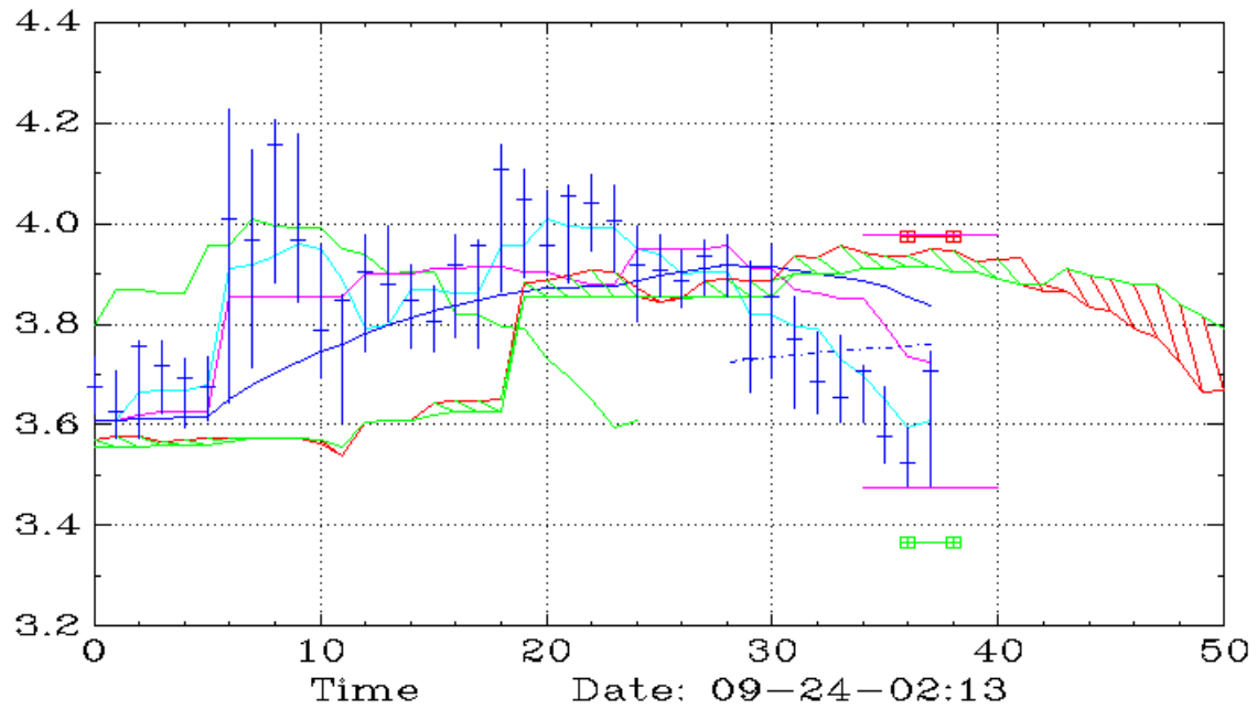
GNPX (10,Ichimoku)
