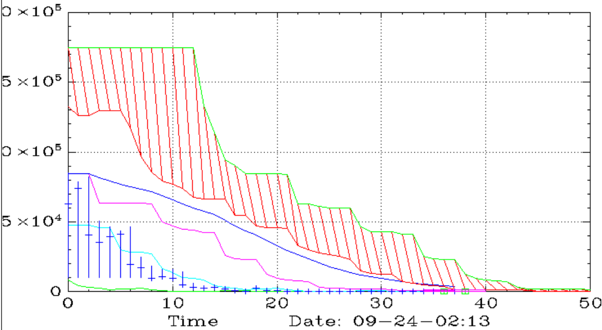
GNPX (Monthly,Ichimoku)
