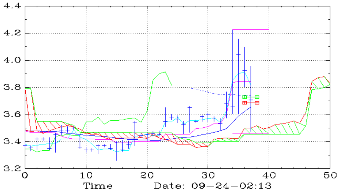
GNPX (90,Ichimoku)
