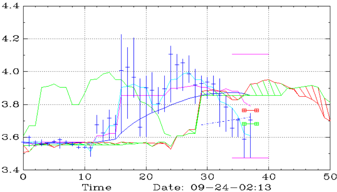
GNPX (15,Ichimoku)
