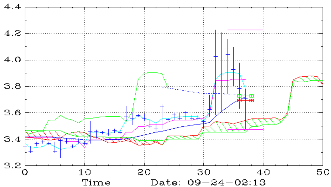
GNPX (60,Ichimoku)
