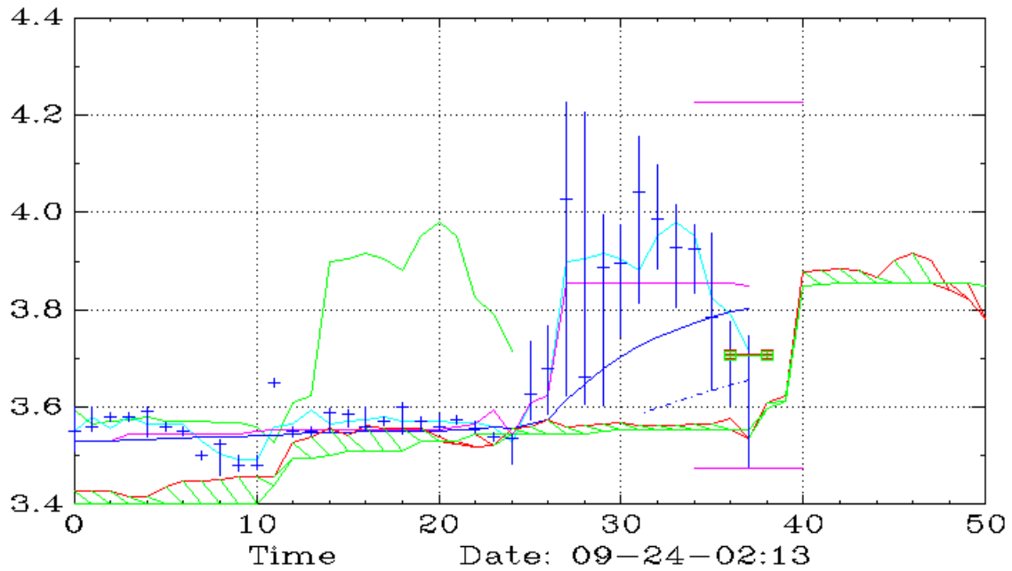
GNPX (30,Ichimoku)
