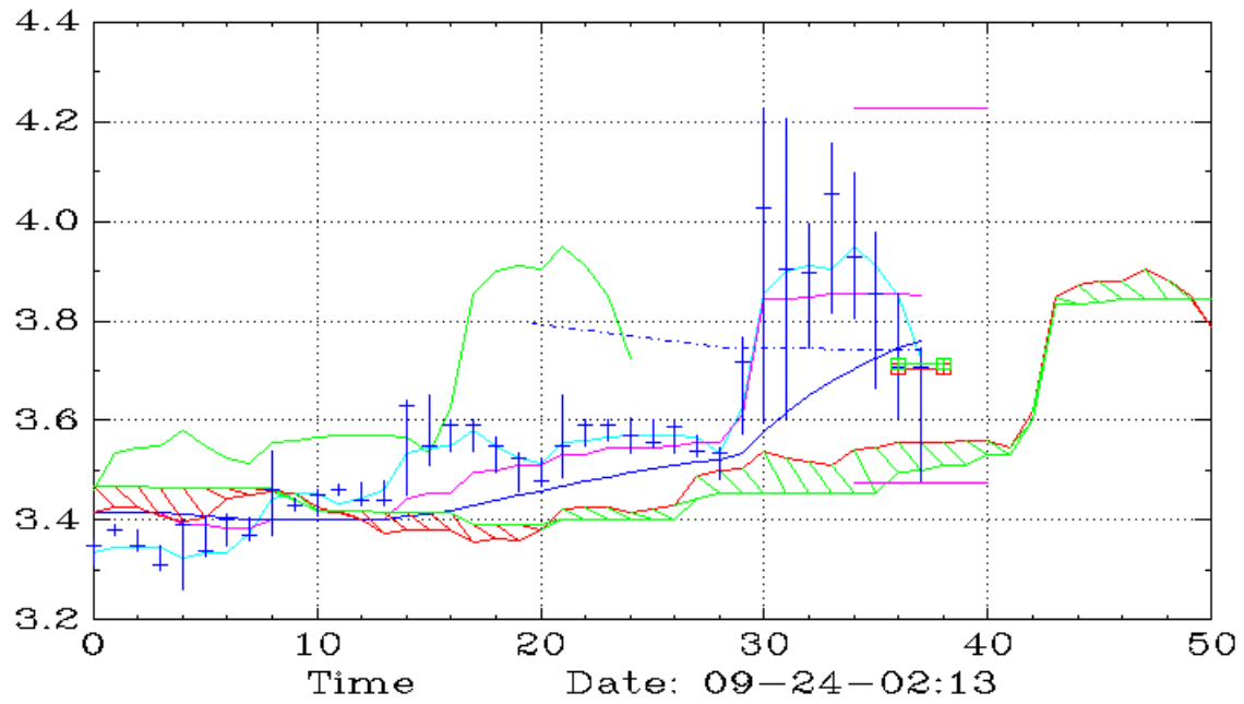
GNPX (45,Ichimoku)
