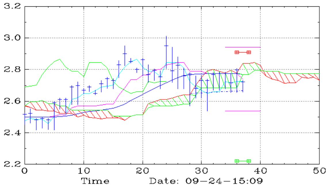
HKIT (10,Ichimoku)
