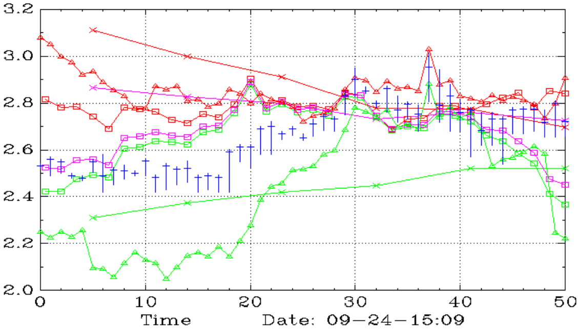
HKIT (90,15,10)
