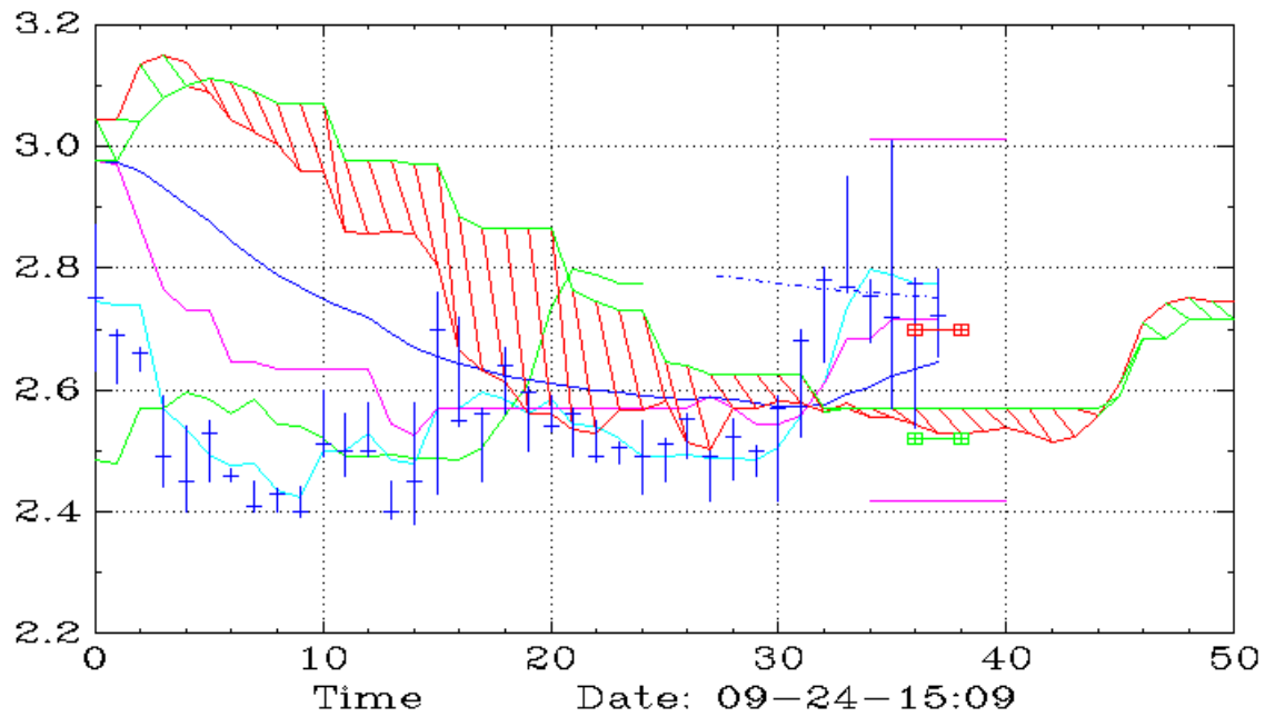
HKIT (90,Ichimoku)
