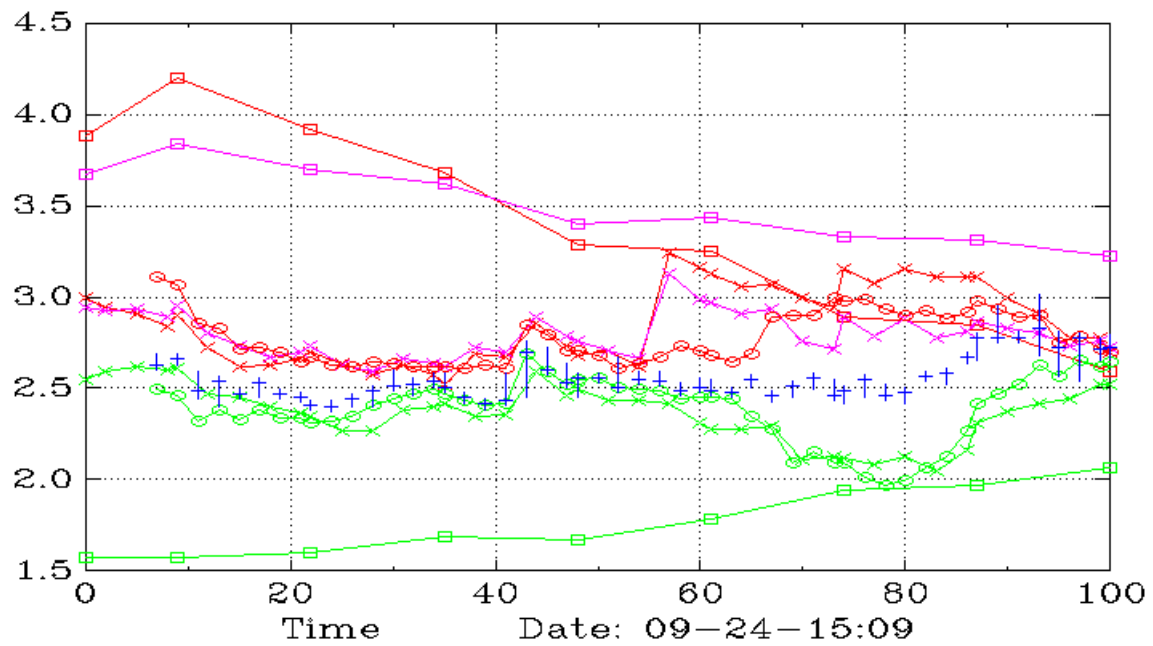
HKIT (Daily,90,60)
