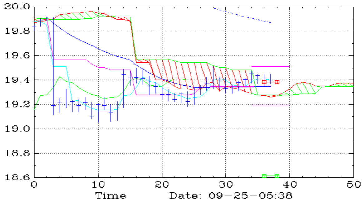
IAG (10,Ichimoku)
