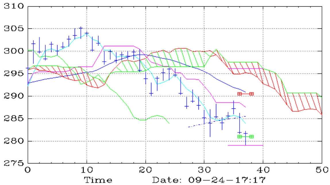
IWM (Daily,Ichimoku)
