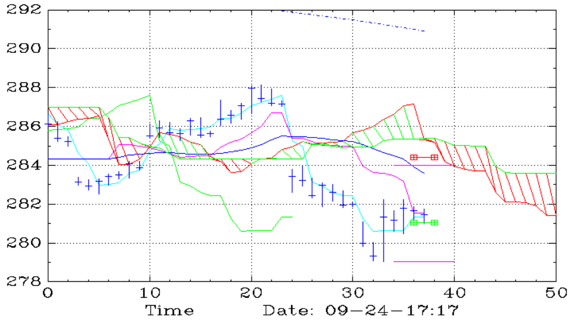
IWM (60,Ichimoku)
