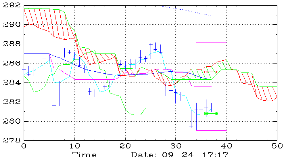
IWM (90,Ichimoku)
