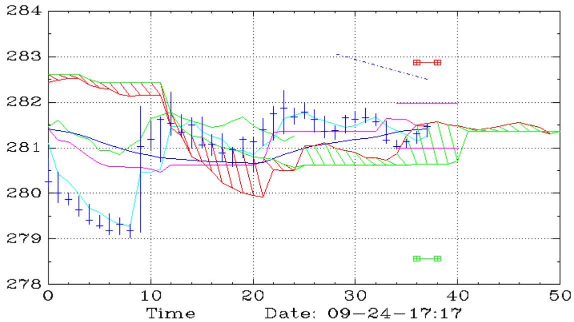
IWM (10,Ichimoku)
