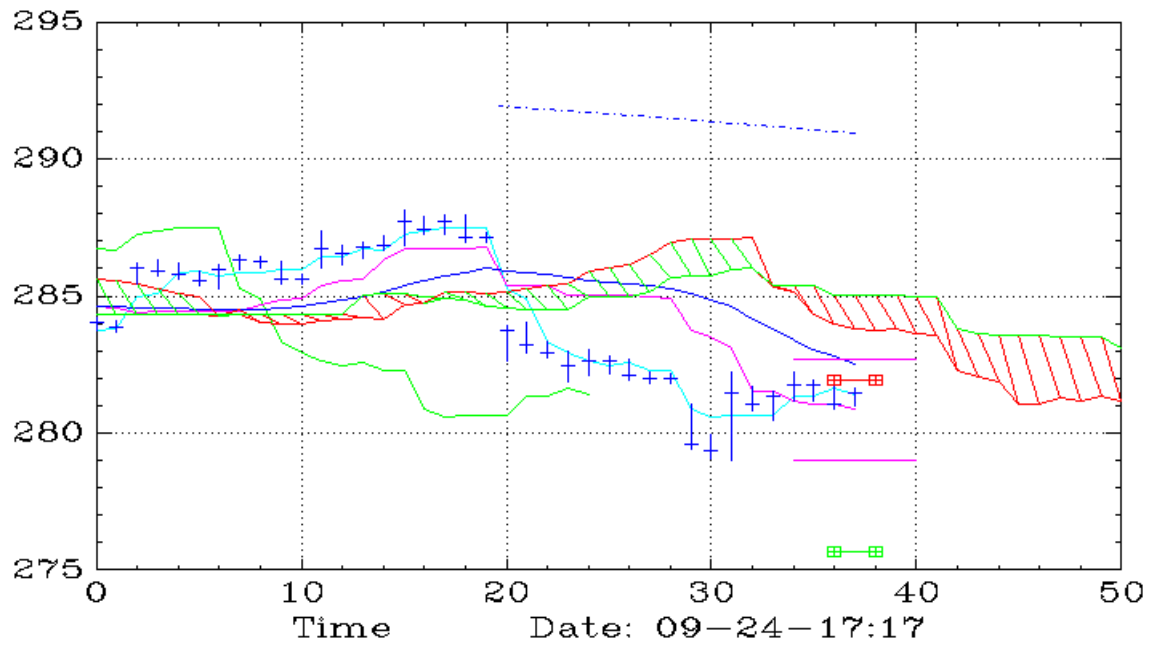
IWM (45,Ichimoku)
