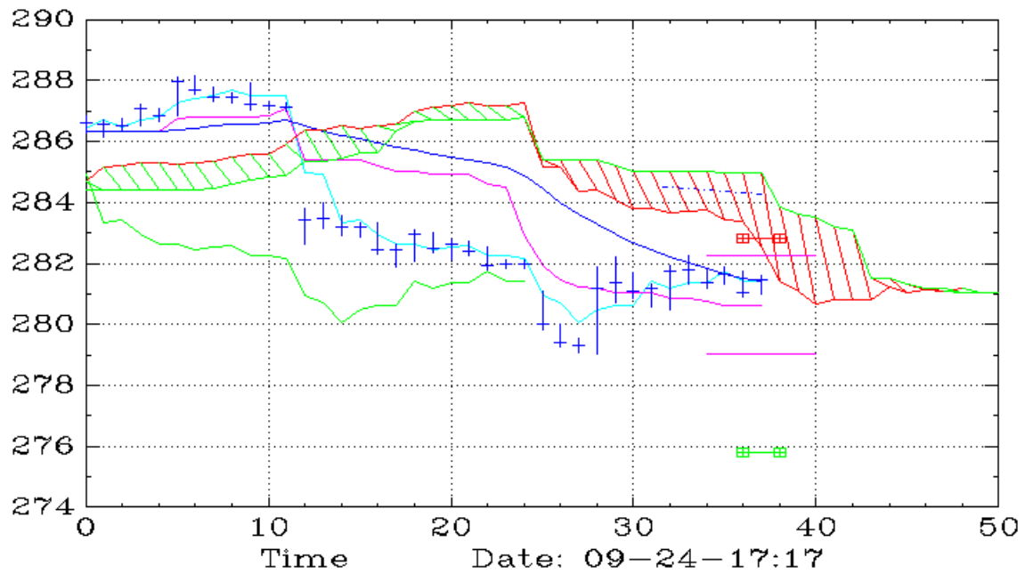
IWM (30,Ichimoku)
