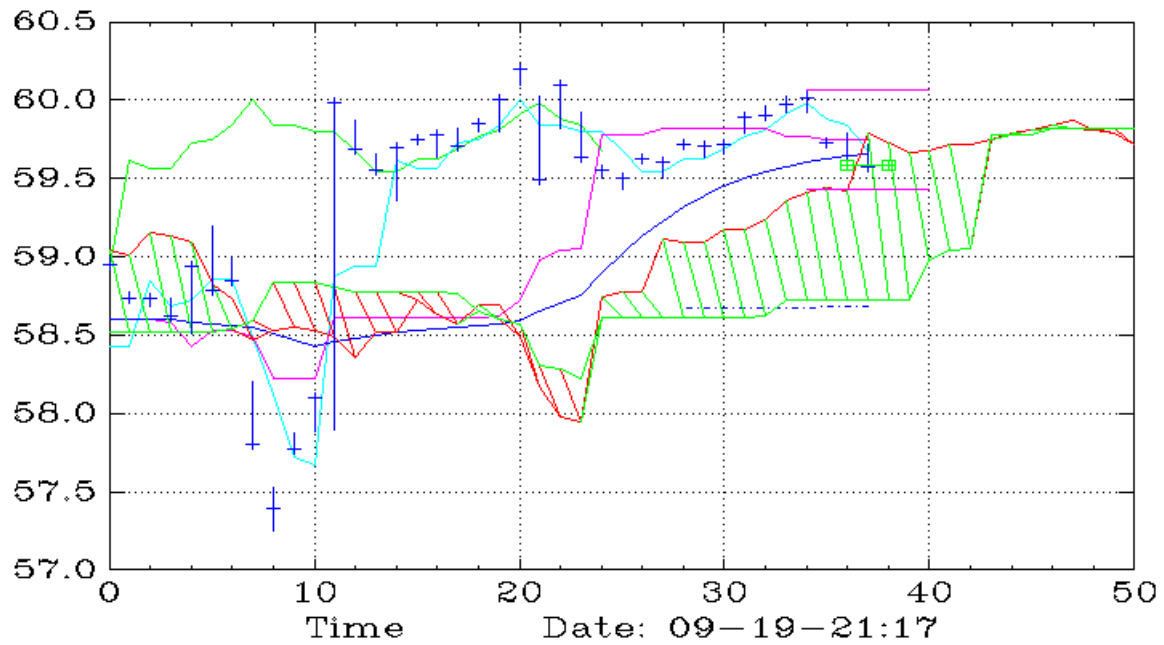
MAGX (10,Ichimoku)
