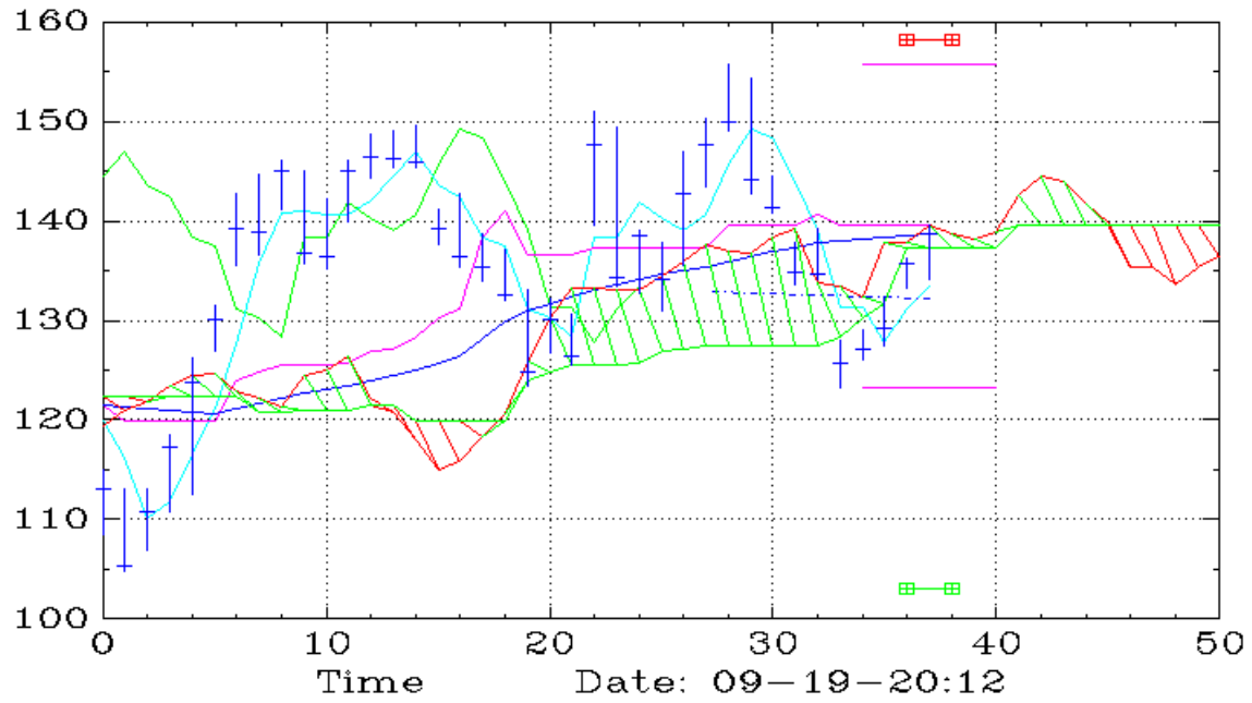
NVDU (Daily,Ichimoku)
