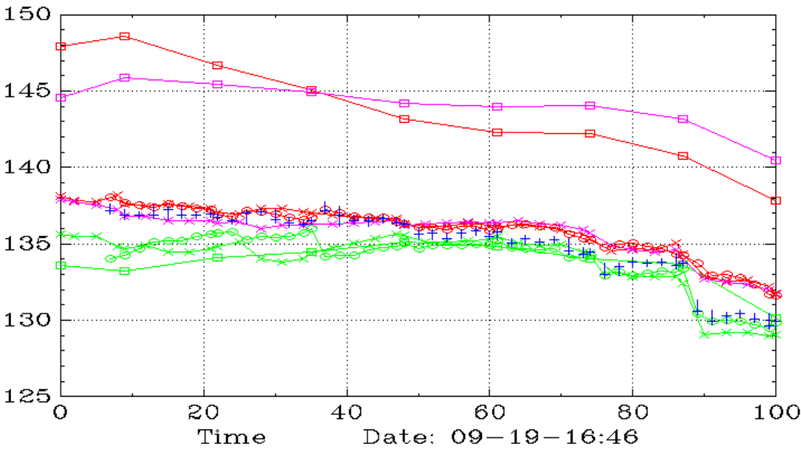
PEP (Daily,90,60)
