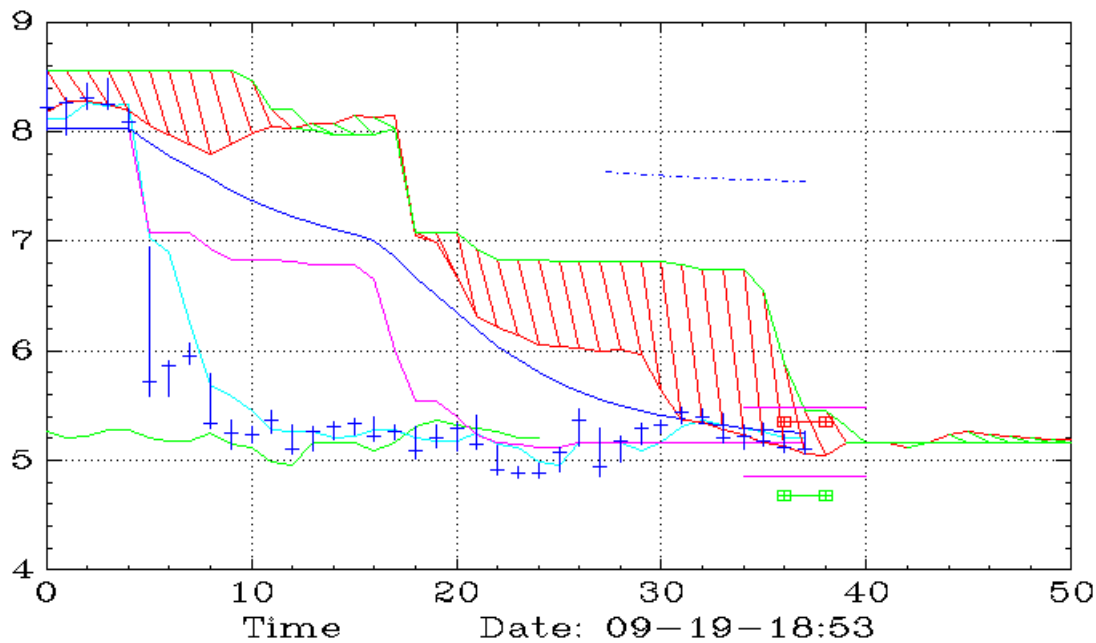
PLTD (Daily,Ichimoku)
