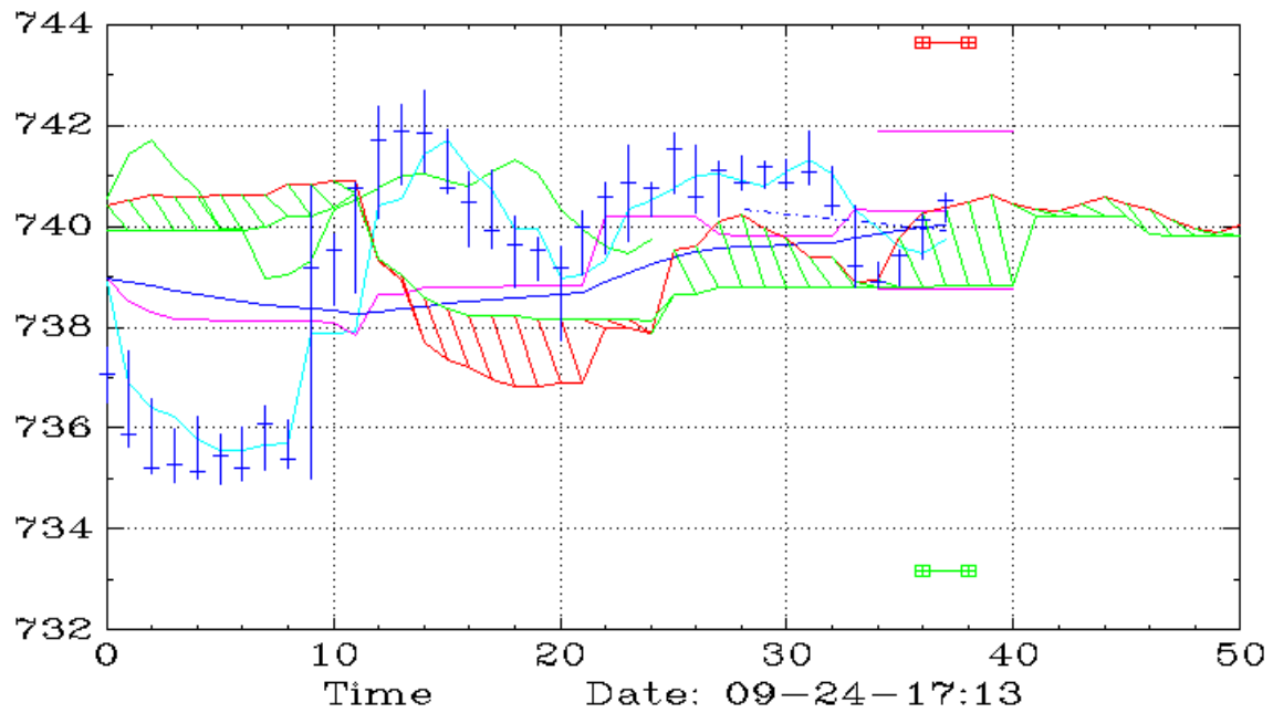
QQQ (10,Ichimoku)
