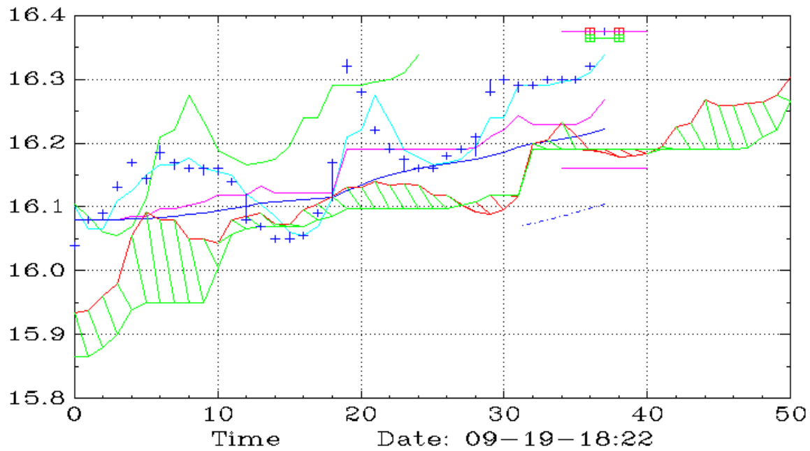
REK (30,Ichimoku)
