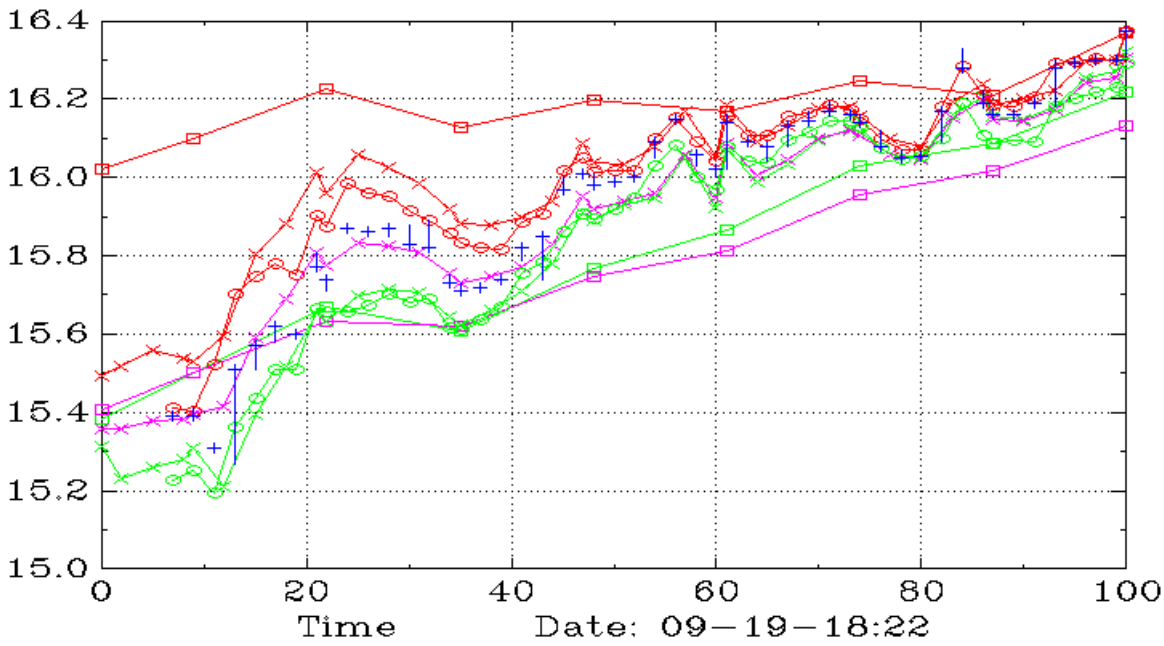
REK (Daily,90,60)
