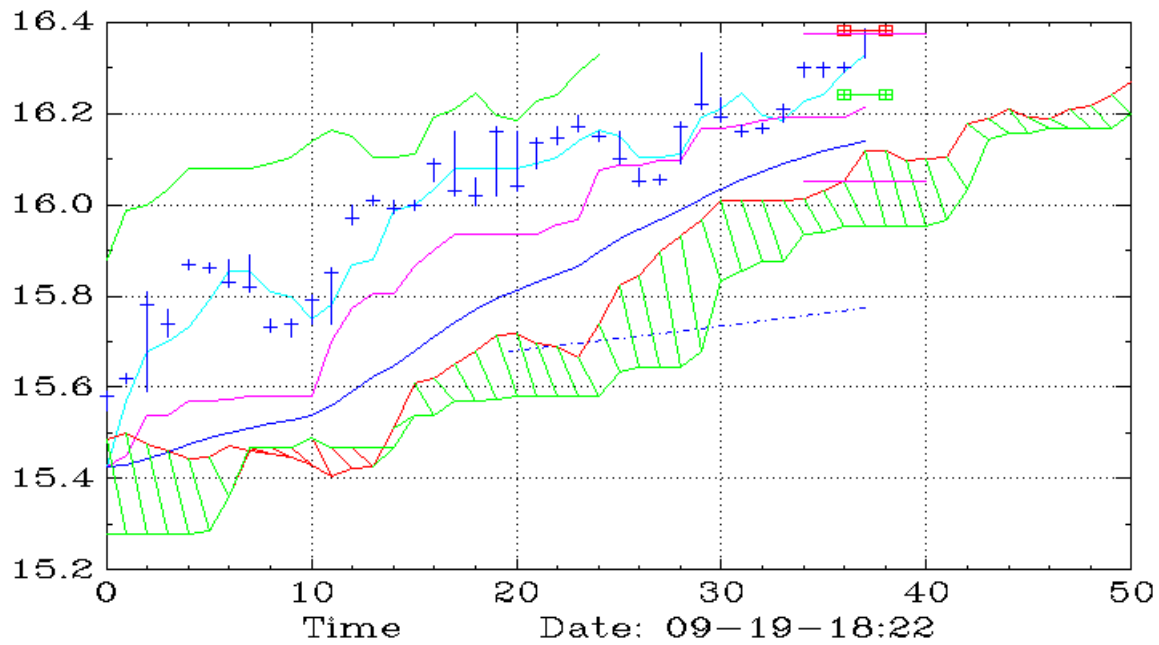
REK (45,Ichimoku)
