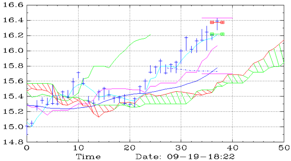
REK (Daily,Ichimoku)
