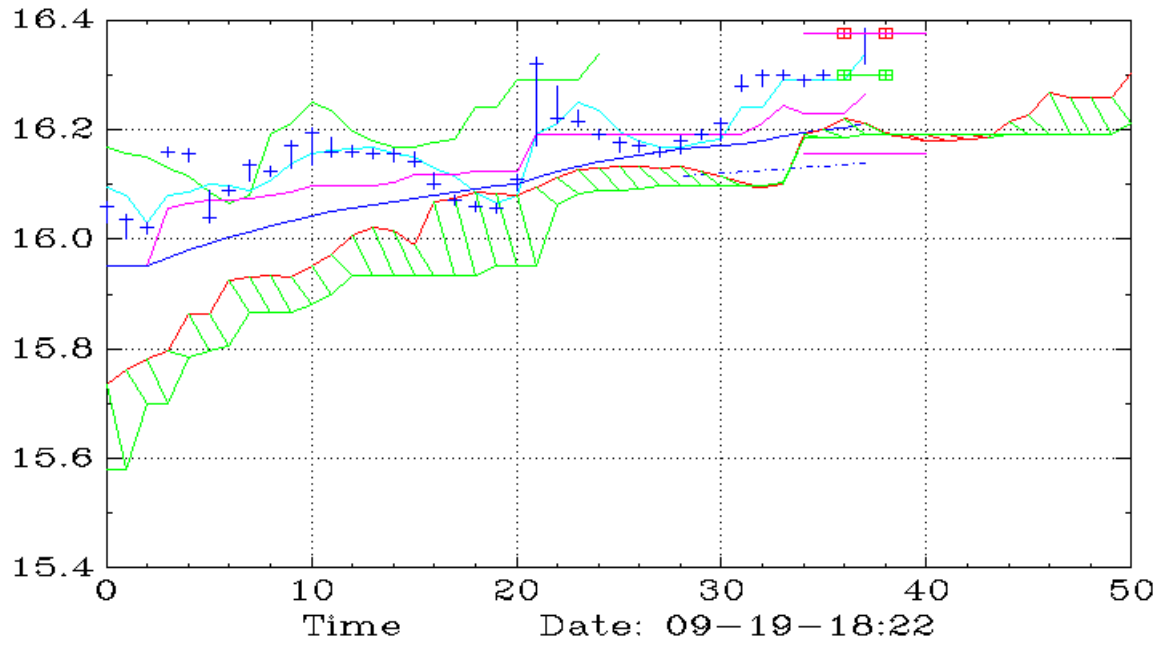
REK (10,Ichimoku)
