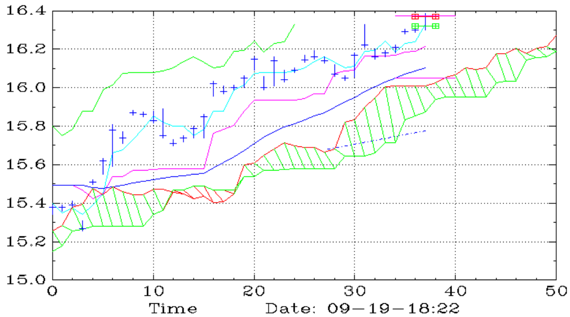
REK (90,Ichimoku)
