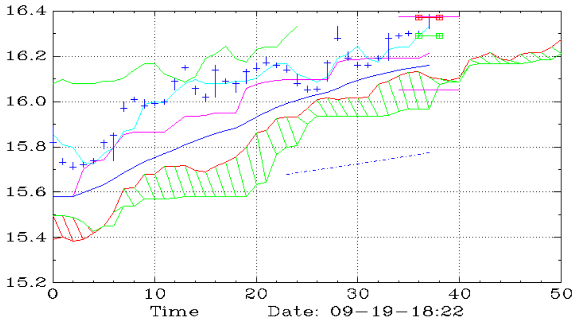
REK (60,Ichimoku)
