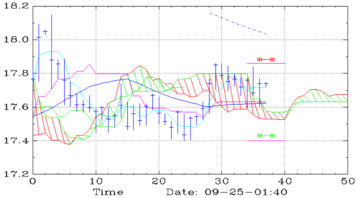
RLAY (10,Ichimoku)
