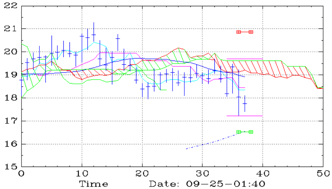
RLAY (Daily,Ichimoku)
