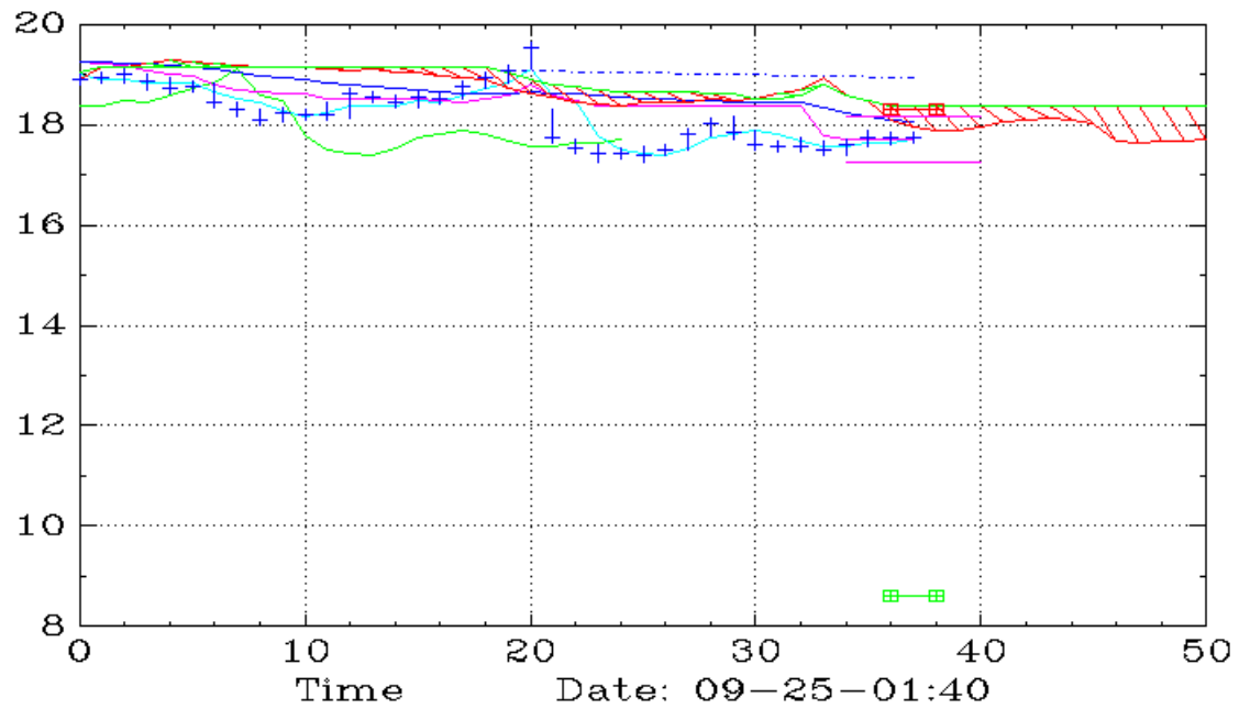
RLAY (45,Ichimoku)
