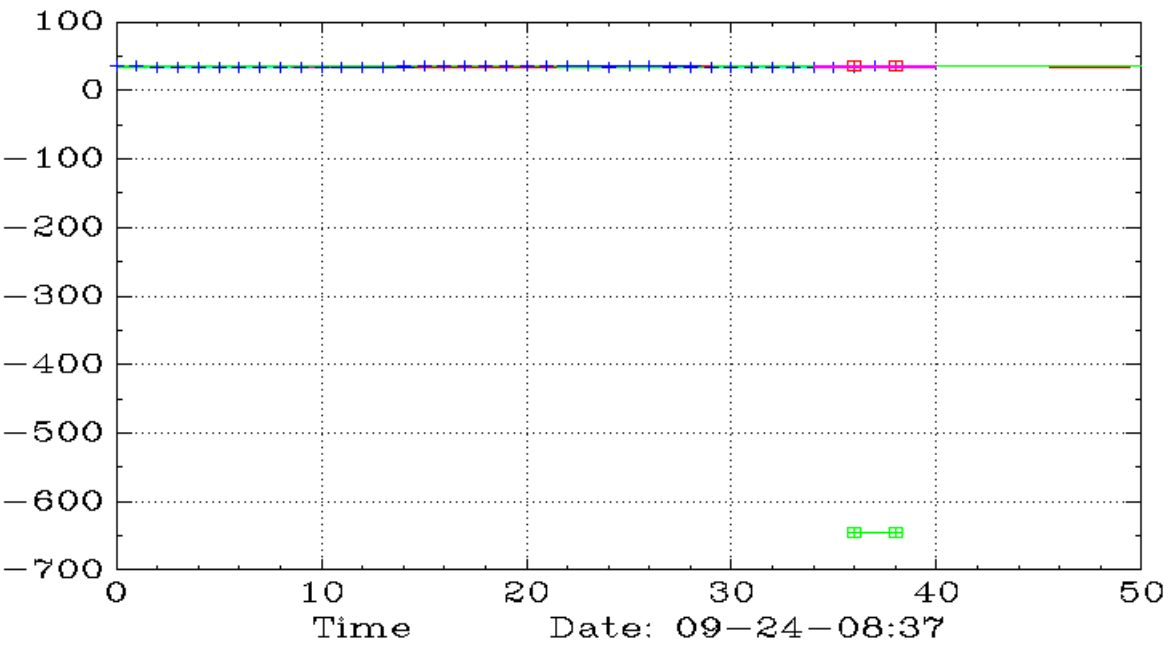
SM (15,Ichimoku)
