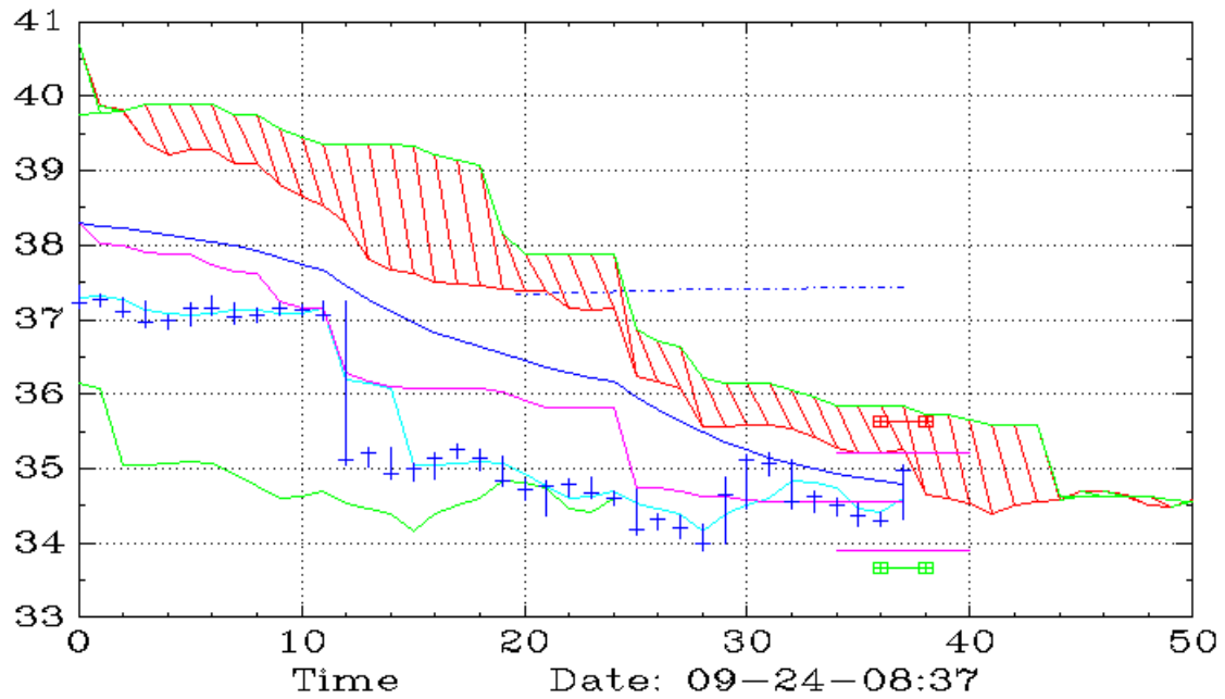
SM (45,Ichimoku)
