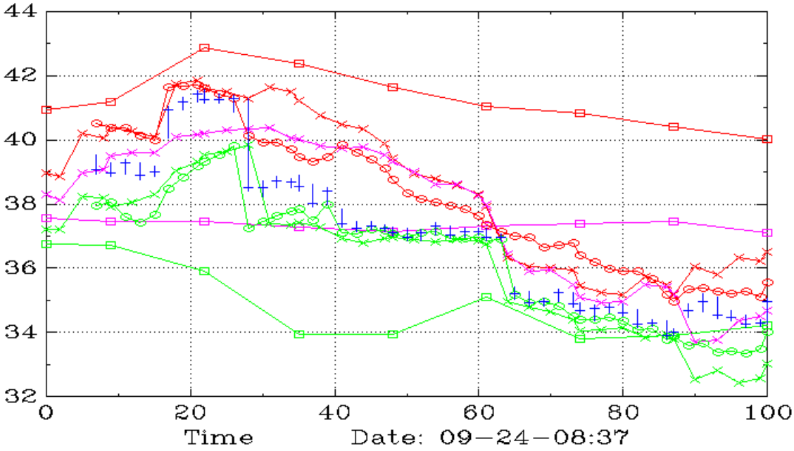
SM (Daily,90,60)
