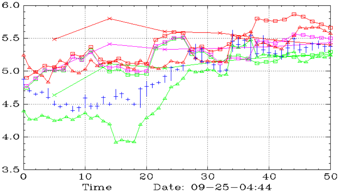
SPRC (90,15,10)
