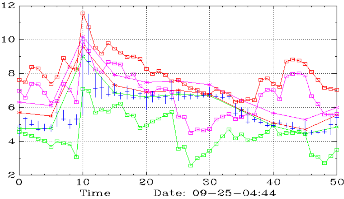
SPRC (Weekly,Daily)
