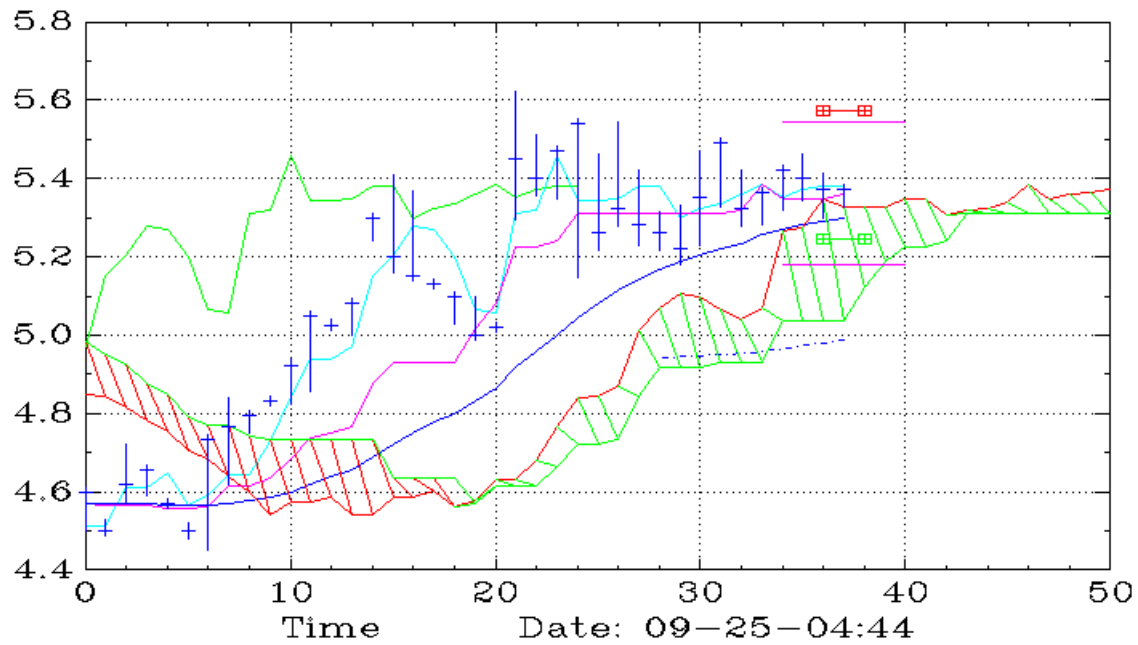
SPRC (10,Ichimoku)
