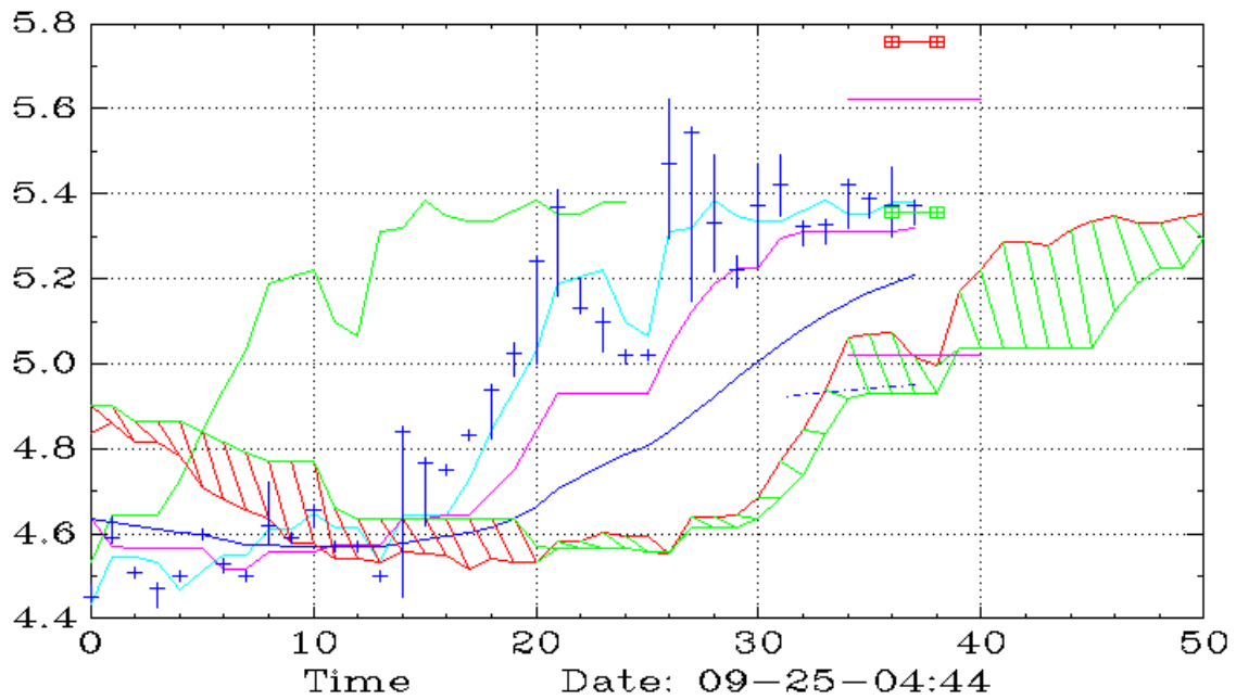
SPRC (30,Ichimoku)
