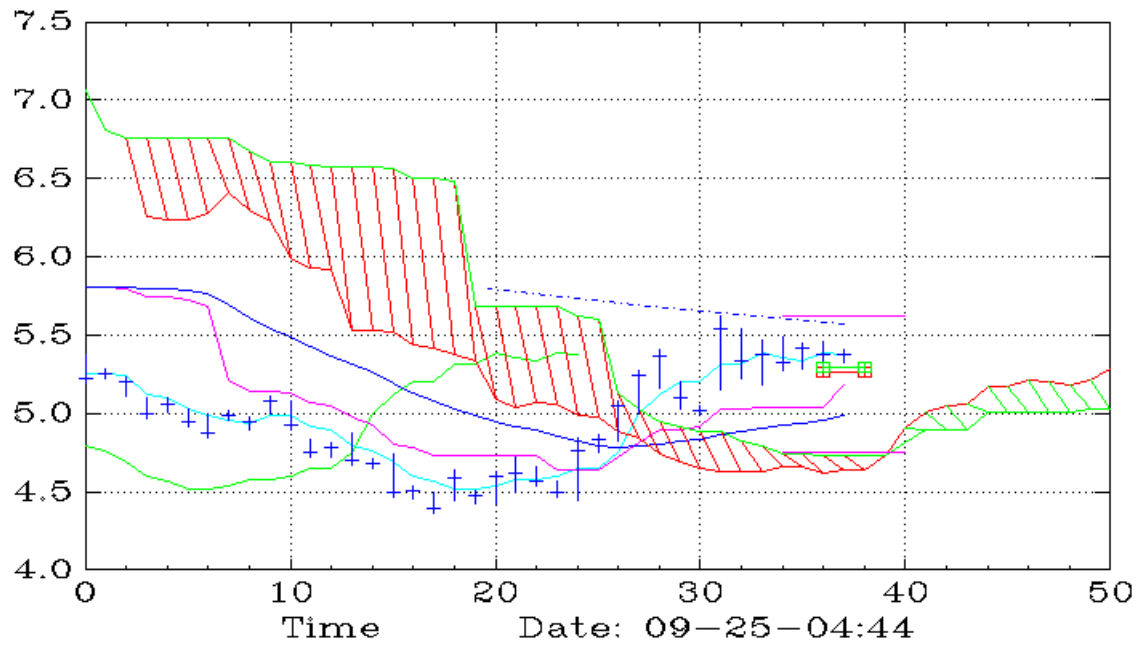
SPRC (45,Ichimoku)
