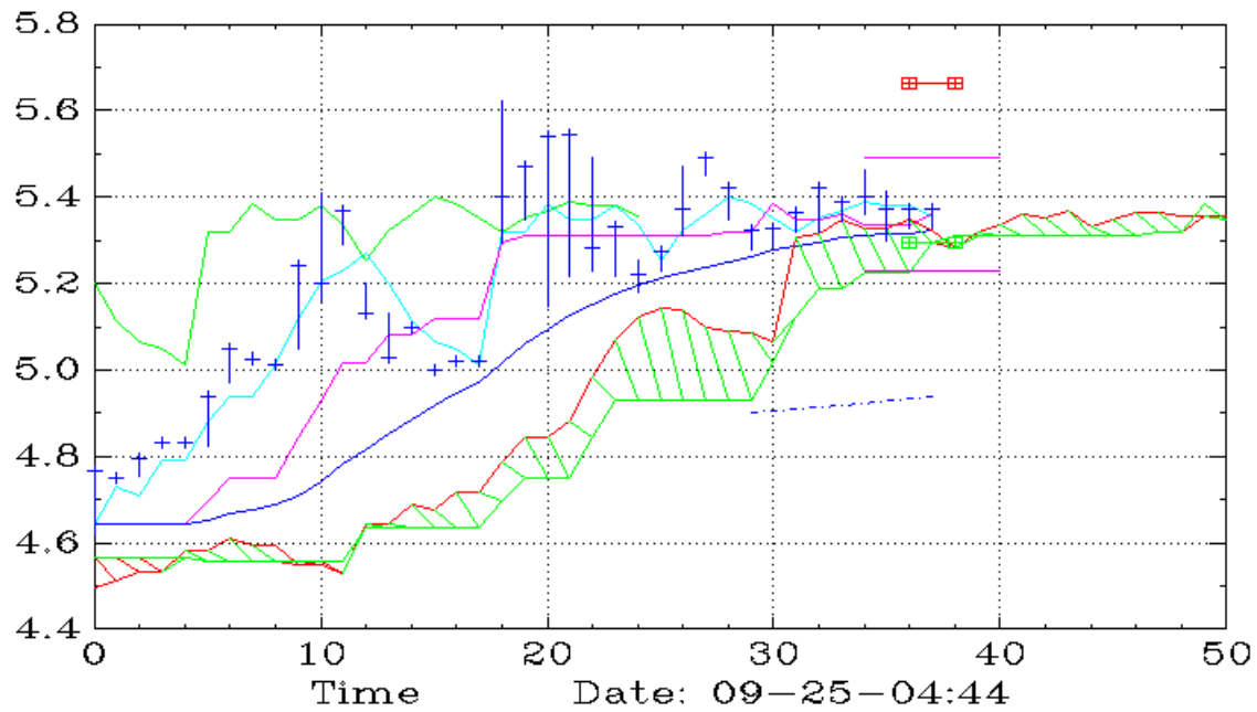
SPRC (15,Ichimoku)
