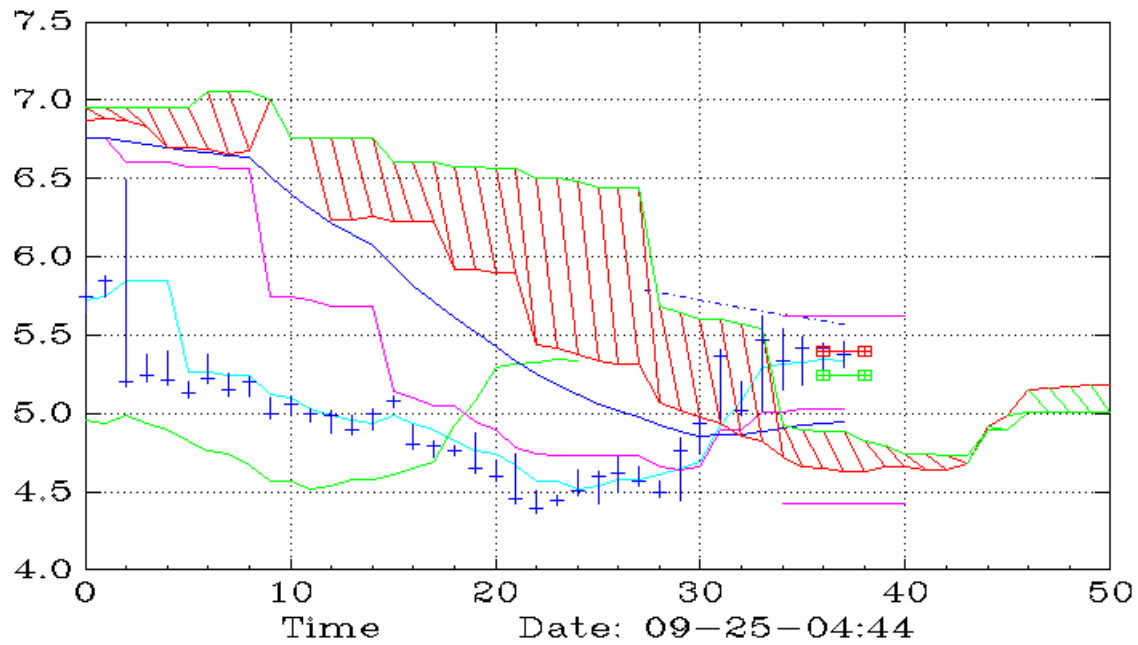
SPRC (90,Ichimoku)
