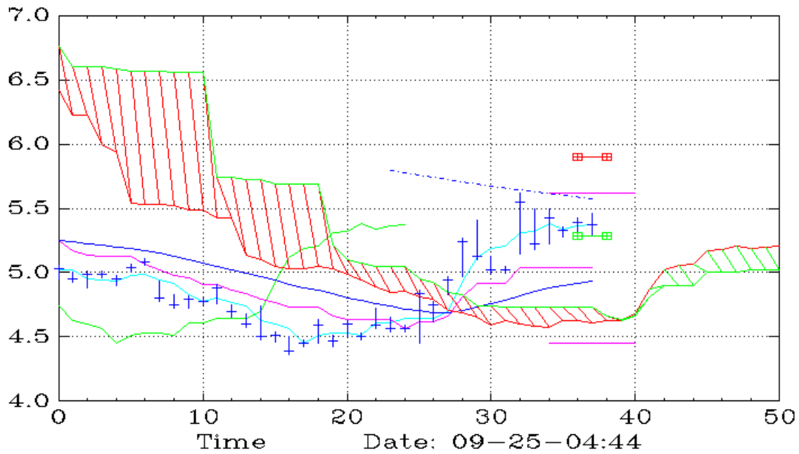
SPRC (60,Ichimoku)
