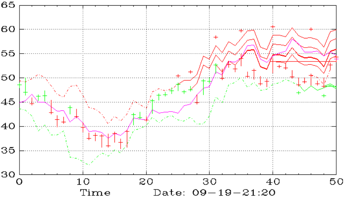
TARK (Daily,SAR)
