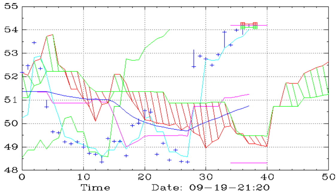
TARK (30,VAP_Ichimoku)
