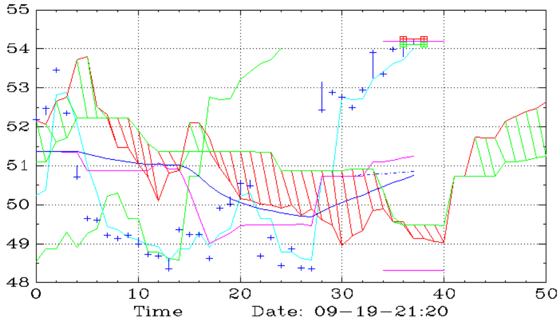
TARK (30,Ichimoku)
