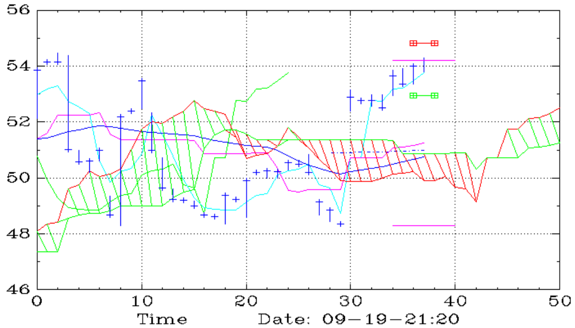
TARK (10,Ichimoku)
