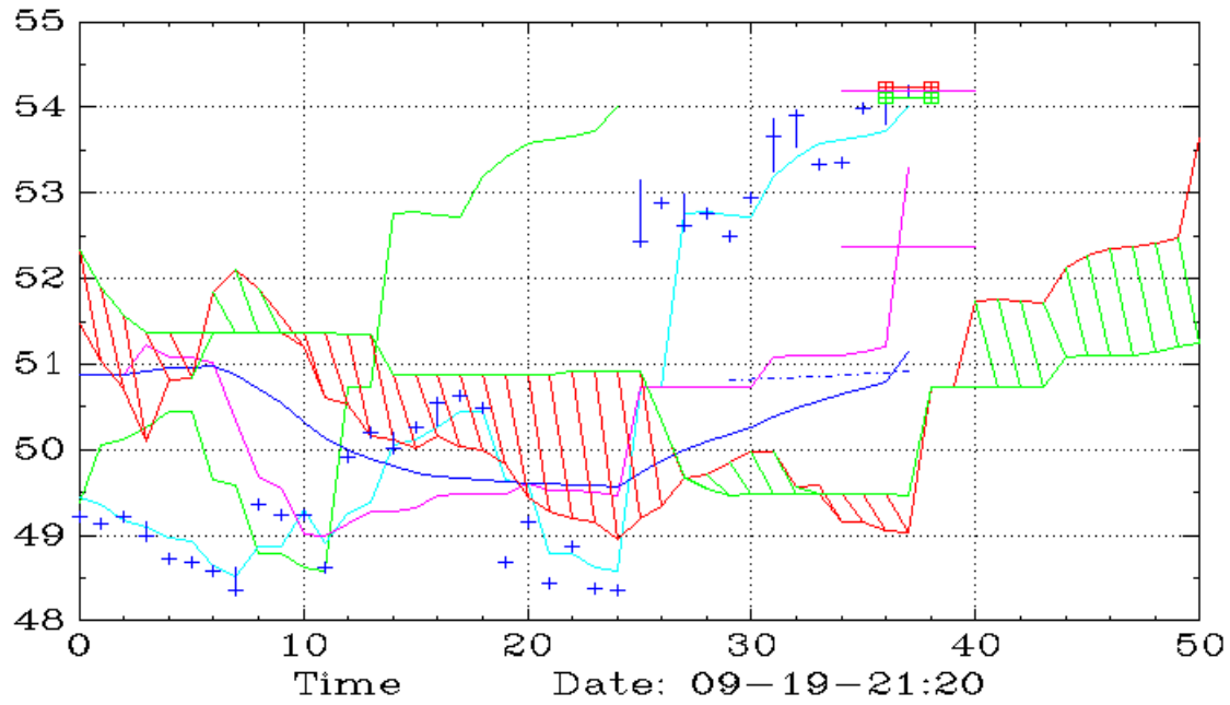
TARK (15,Ichimoku)
