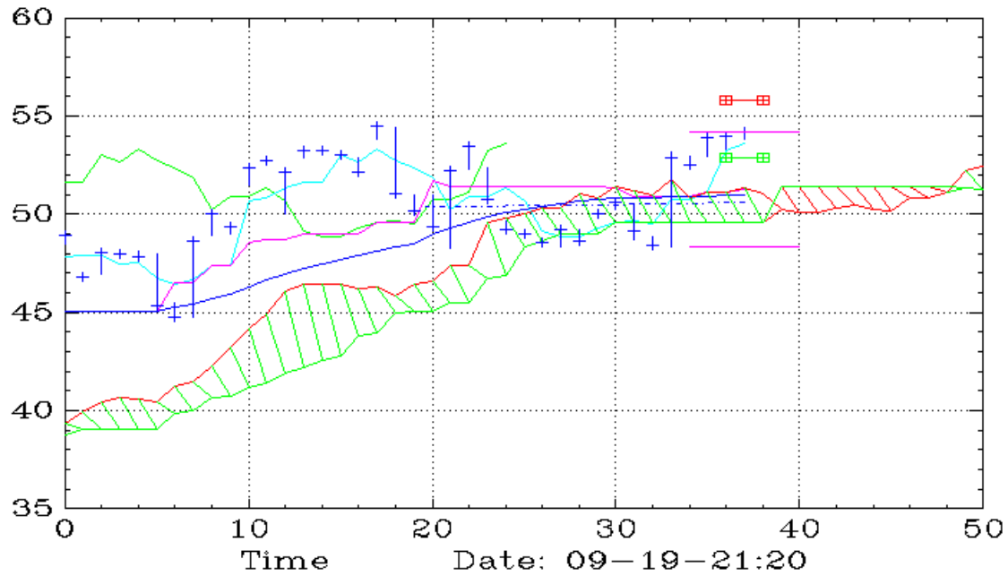
TARK (45,Ichimoku)
