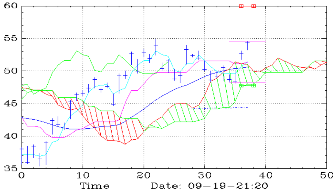
TARK (Daily,Ichimoku)
