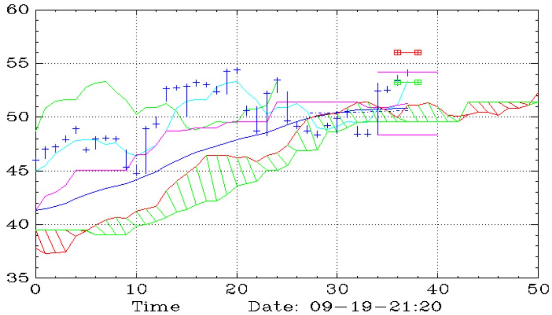
TARK (90,Ichimoku)
