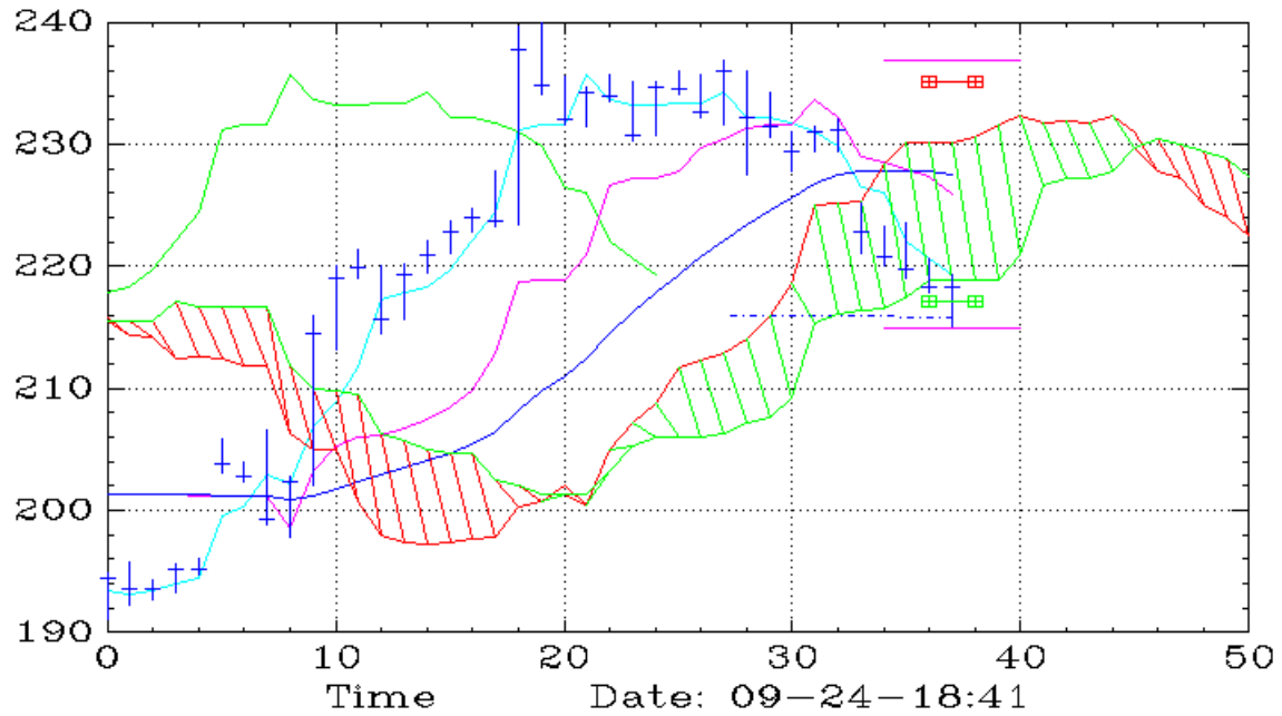
TSEM (90,Ichimoku)
