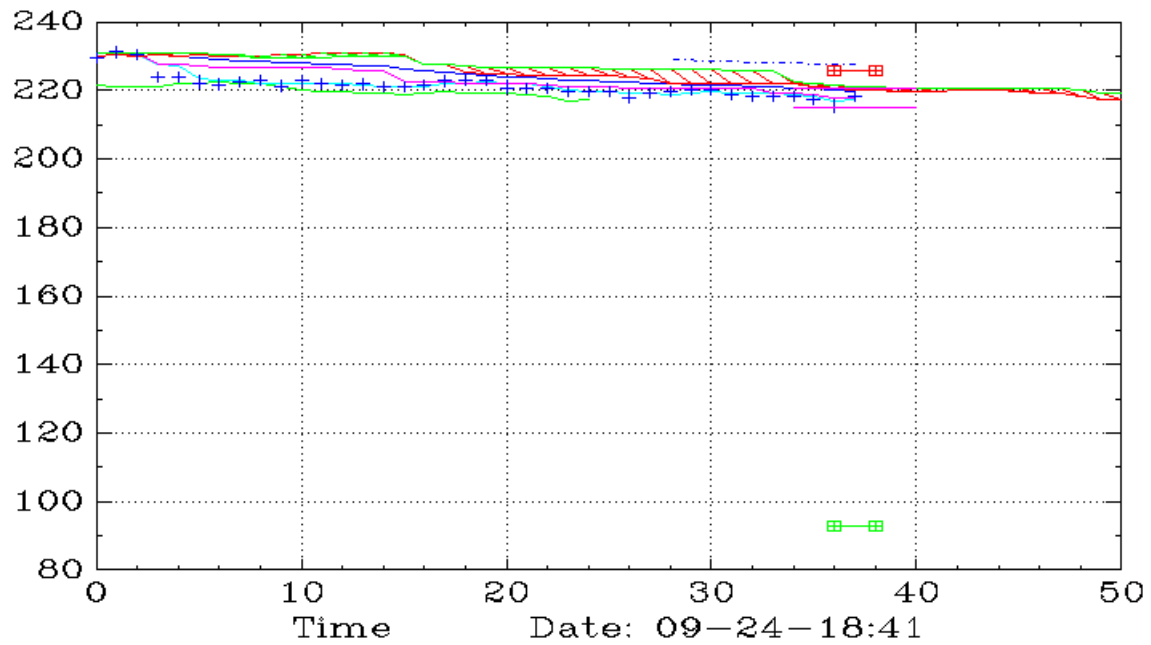
TSEM (10,Ichimoku)
