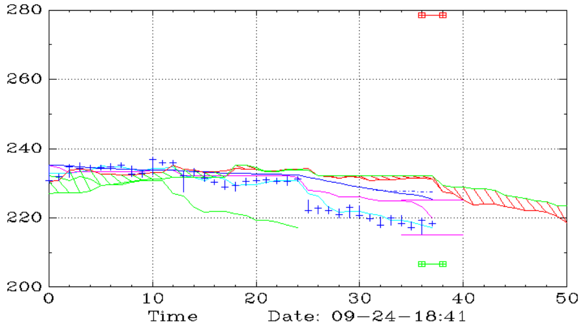
TSEM (30,Ichimoku)
