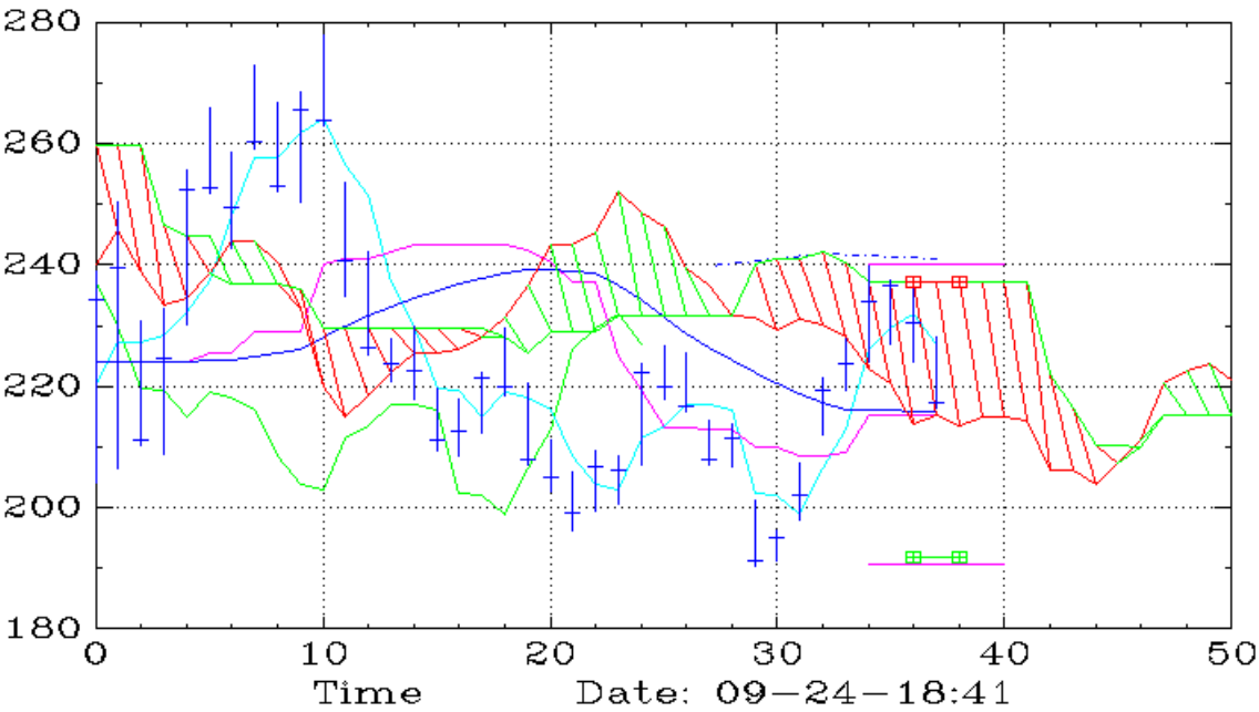
TSEM (Daily,Ichimoku)
