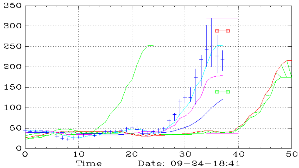
TSEM (Monthly,Ichimoku)
