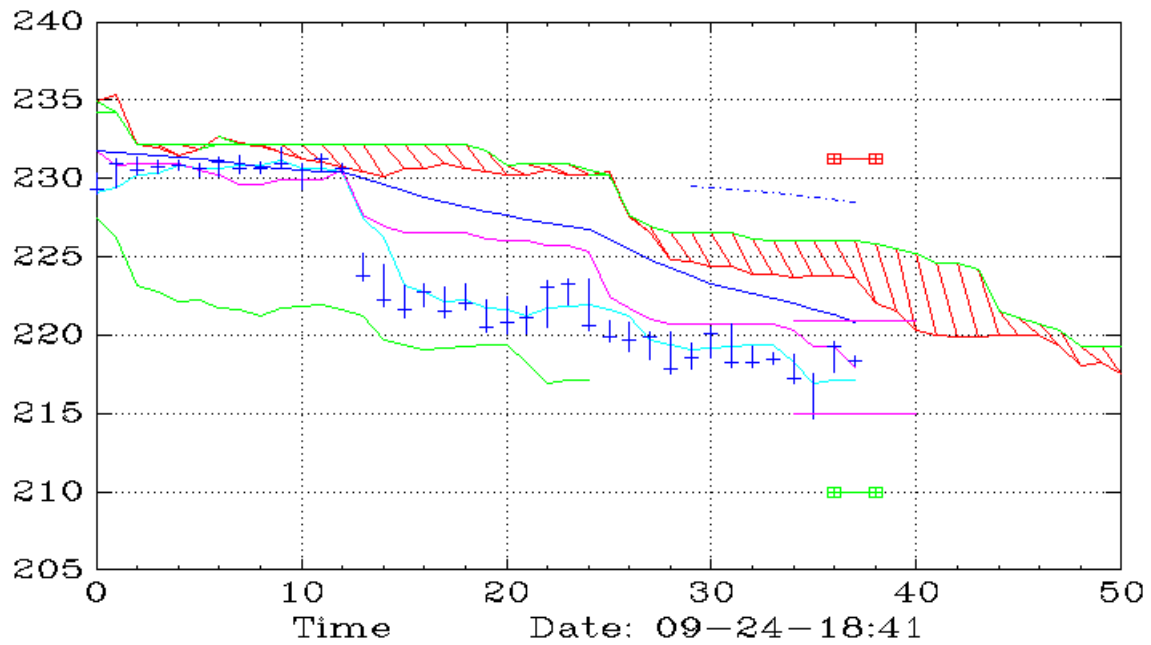
TSEM (15,Ichimoku)
