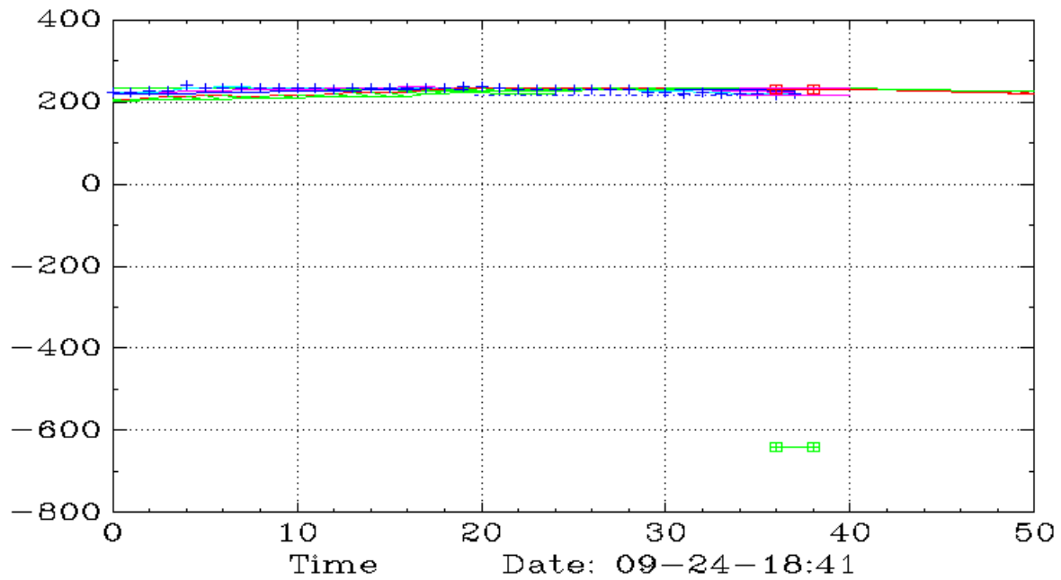
TSEM (45,Ichimoku)
