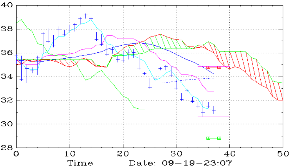
UMDD (Daily,Ichimoku)
