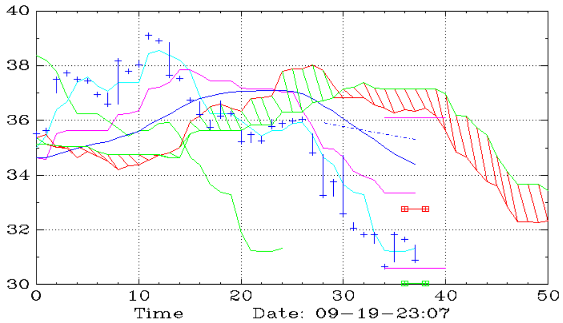
UMDD (10,Ichimoku)
