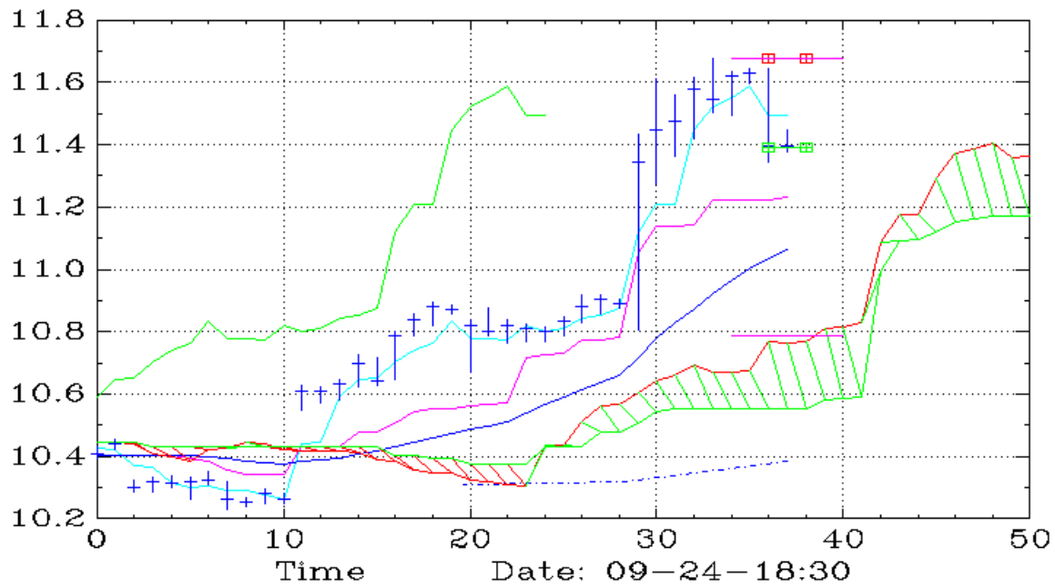
UNG (45,Ichimoku)
