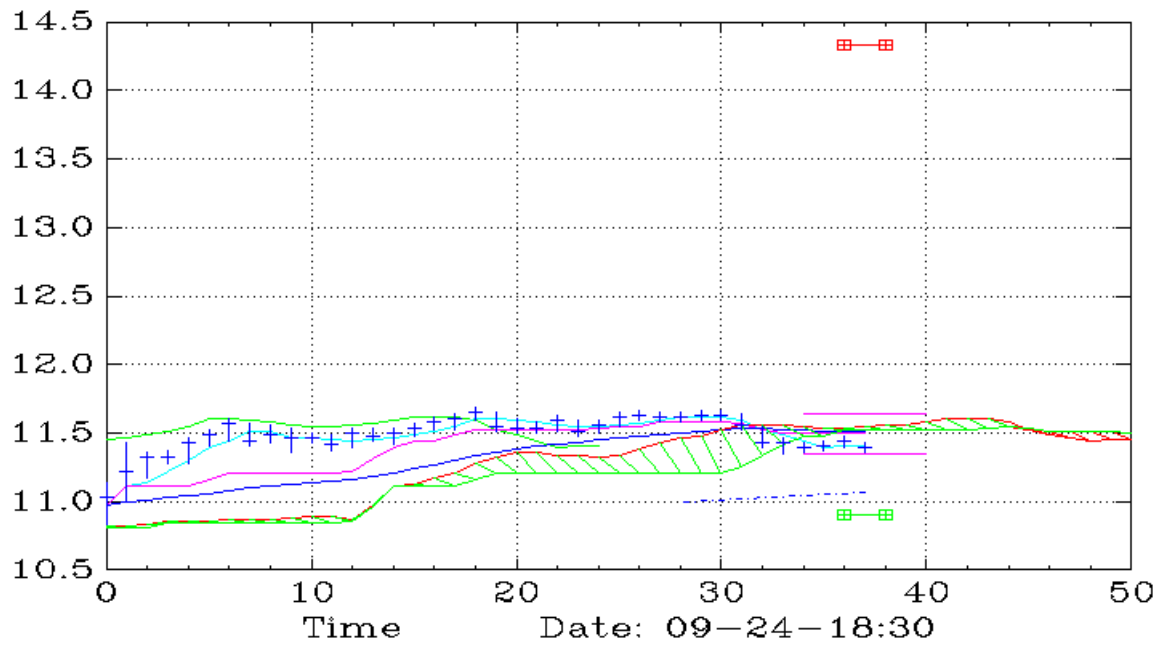
UNG (10,Ichimoku)
