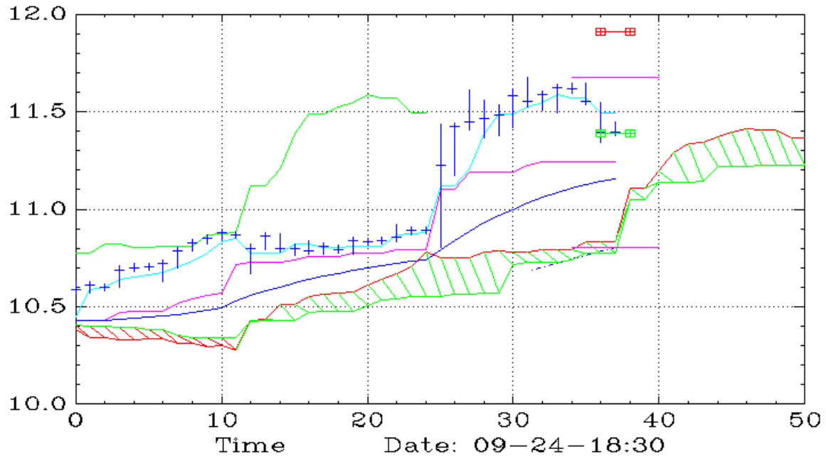
UNG (30,Ichimoku)
