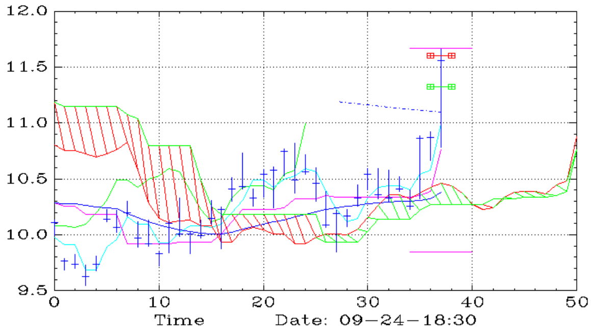
UNG (Daily,Ichimoku)
