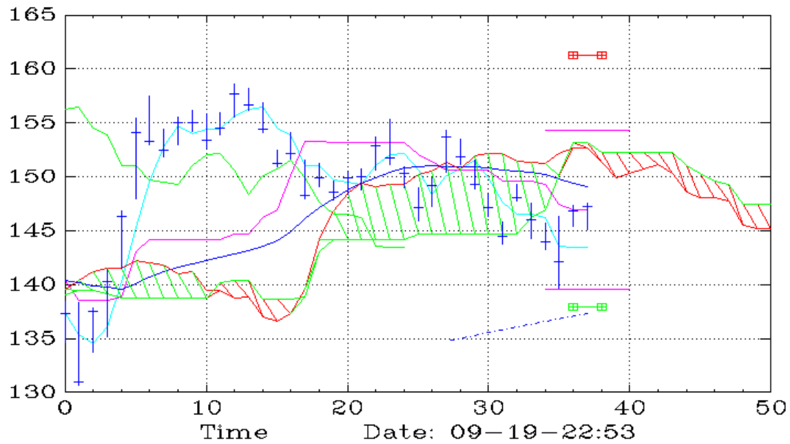
UPRO (Daily,Ichimoku)
