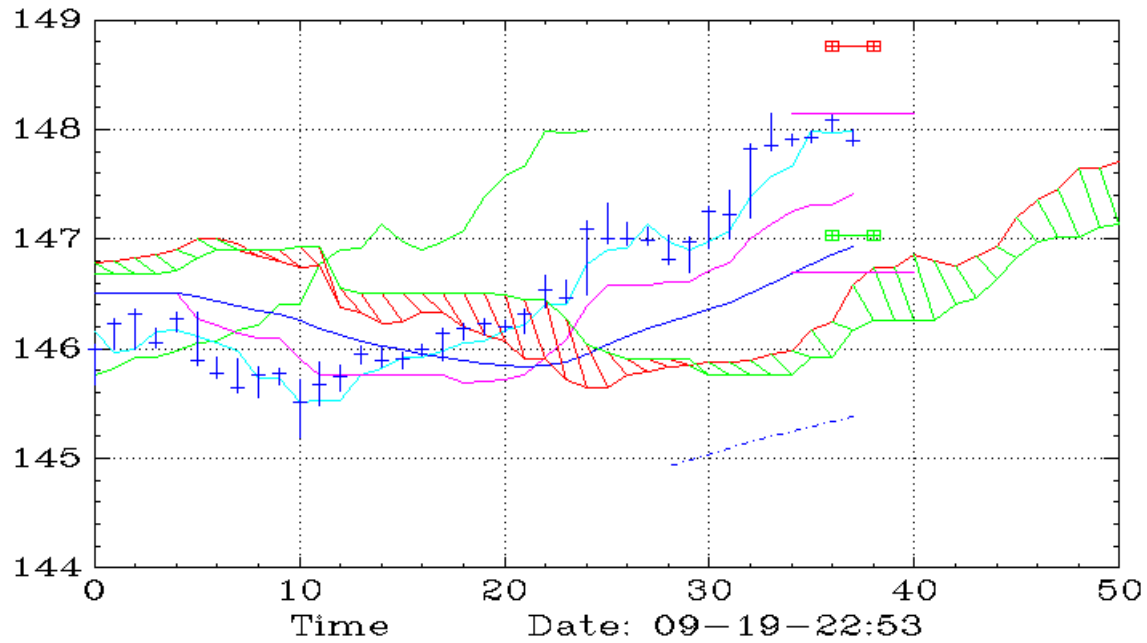
UPRO (10,Ichimoku)
