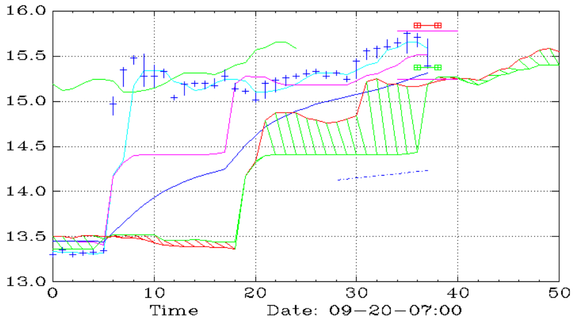
UXRP (10,Ichimoku)
