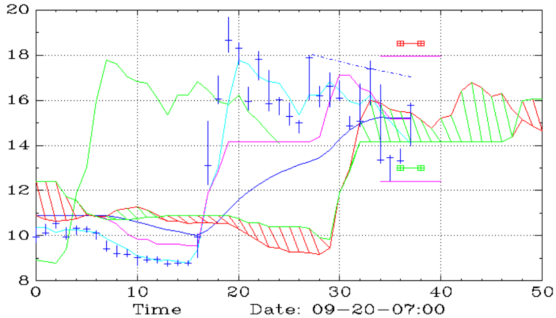
UXRP (Daily,Ichimoku)
