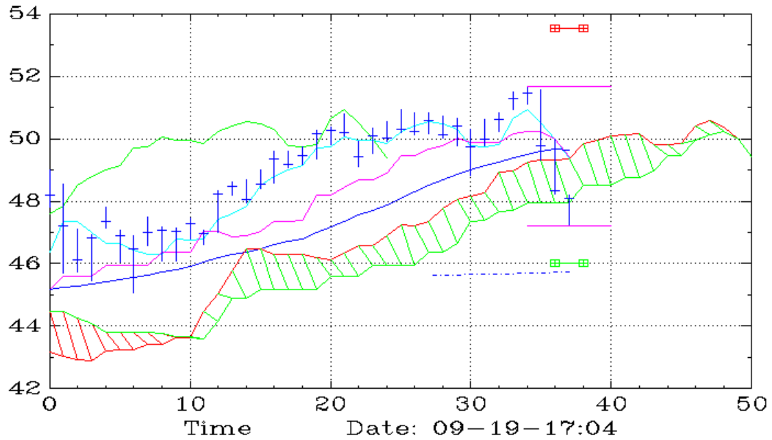
VZ (Daily,Ichimoku)
