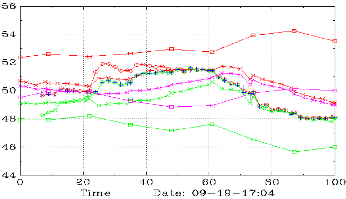
VZ (Daily,90,60)
