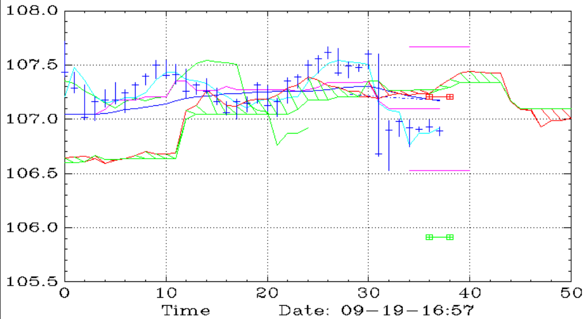
WMT (10,Ichimoku)
