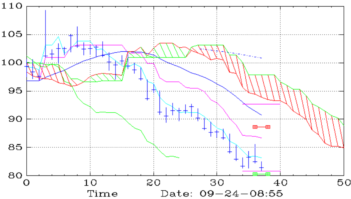
WYNN (Daily,Ichimoku)
