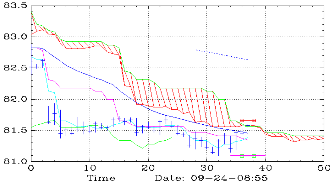
WYNN (10,Ichimoku)
