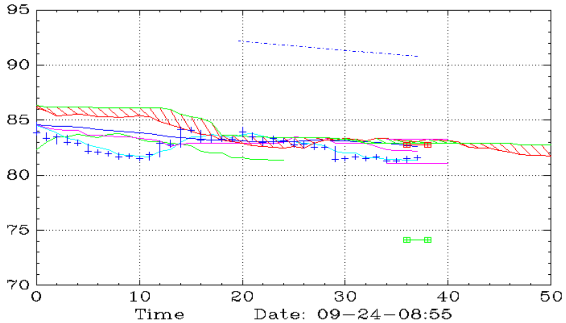
WYNN (45,Ichimoku)
