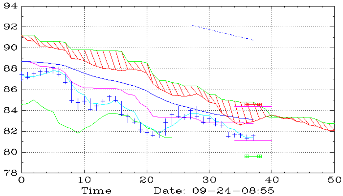
WYNN (90,Ichimoku)
