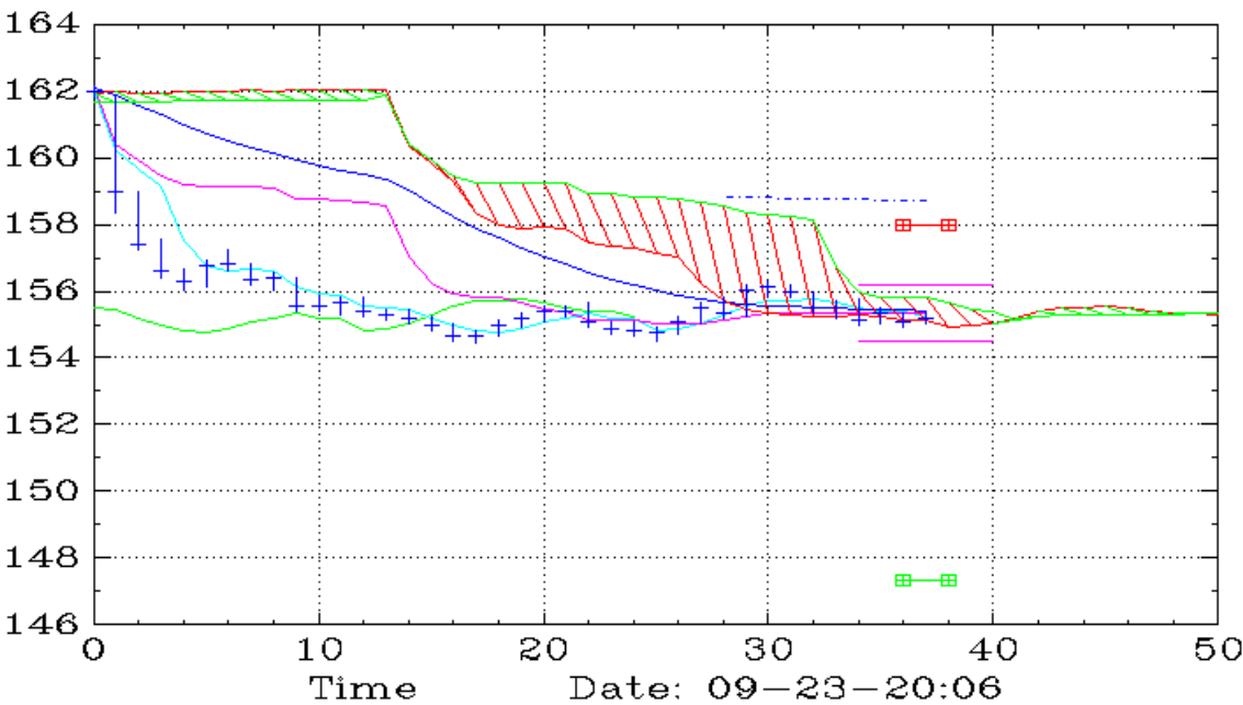
XBI (10,Ichimoku)
