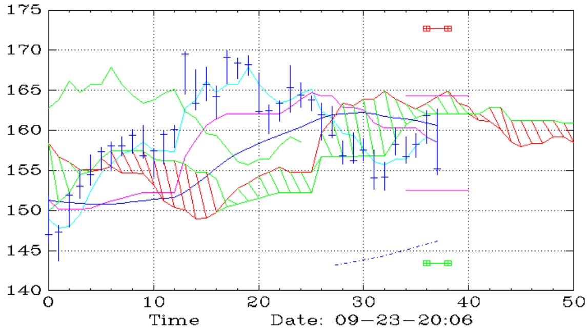
XBI (Daily,Ichimoku)
