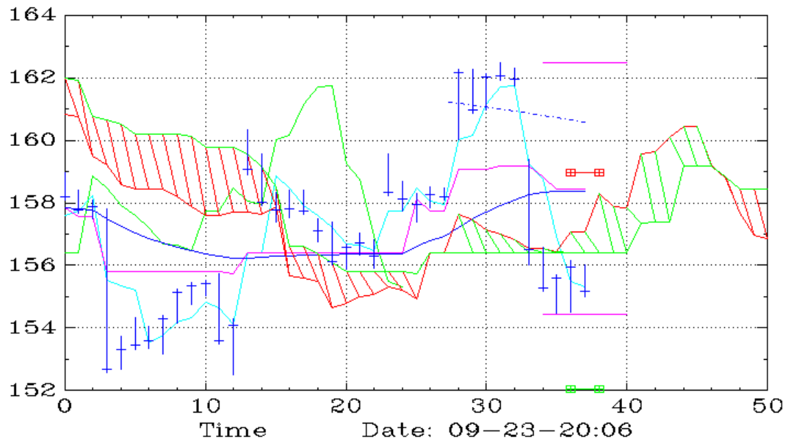
XBI (90,Ichimoku)
