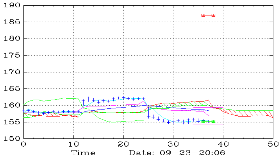
XBI (30,Ichimoku)
