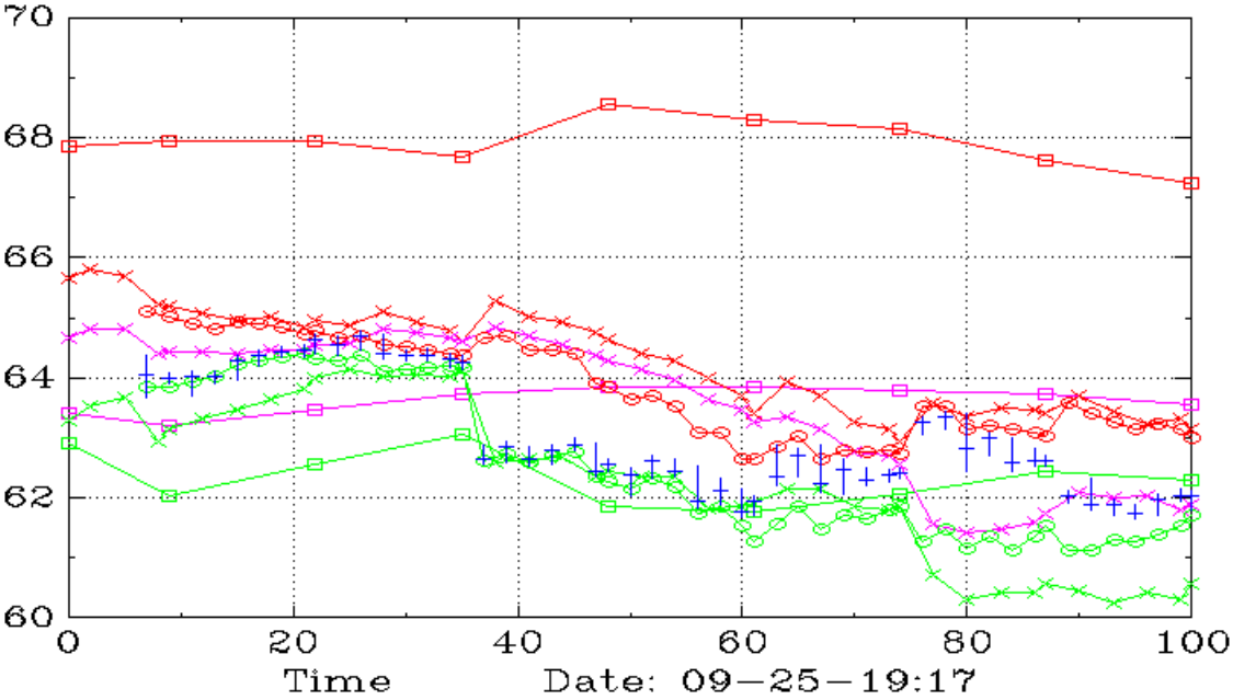
XLE (Daily,90,60)
