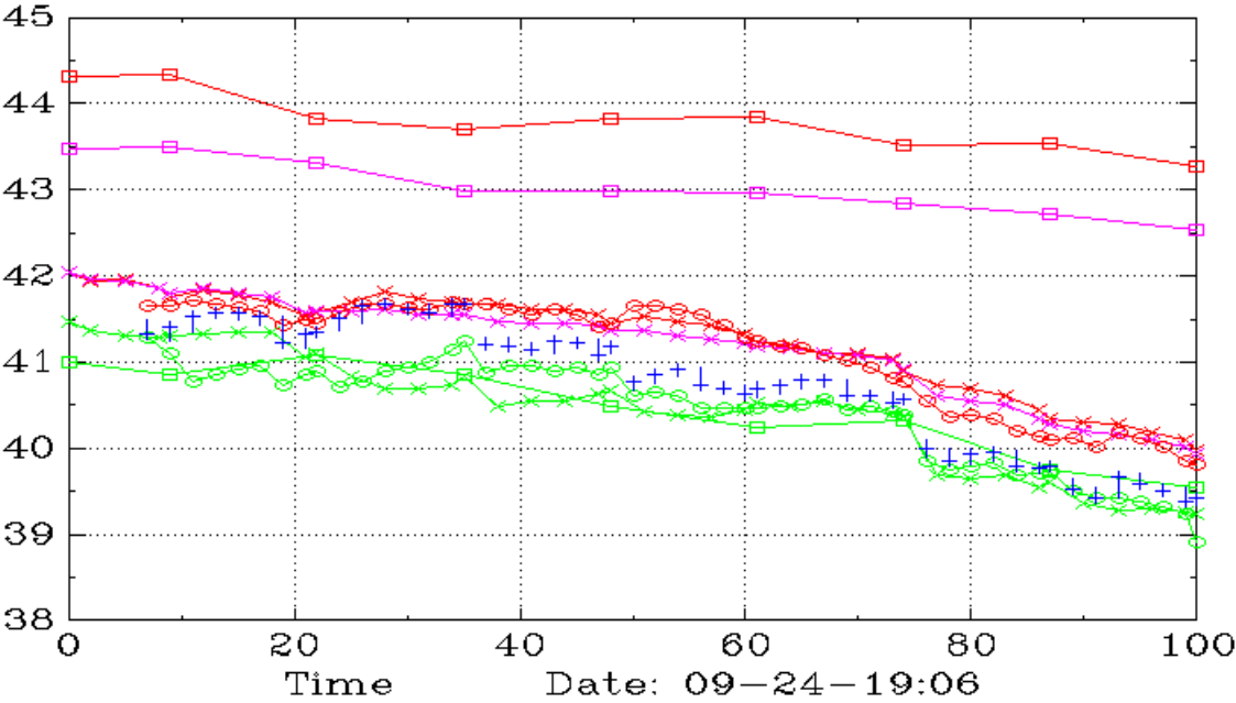
XLU (Daily,90,60)
