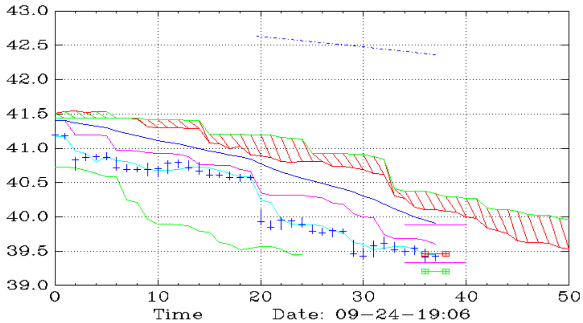
XLU (45,Ichimoku)
