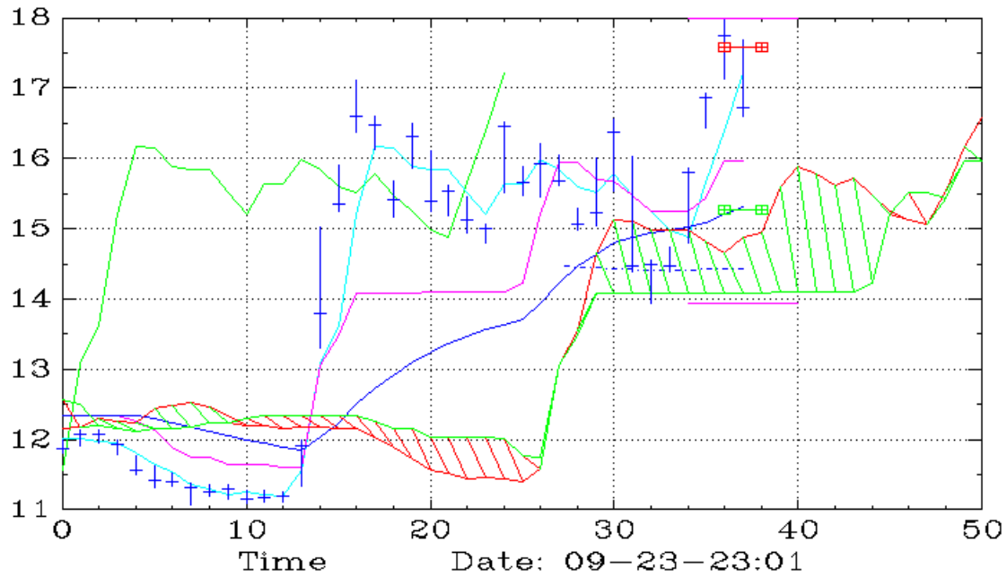
XRP (Daily,Ichimoku)
