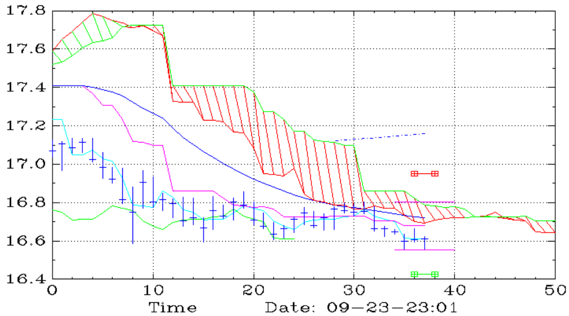
XRP (10,Ichimoku)
